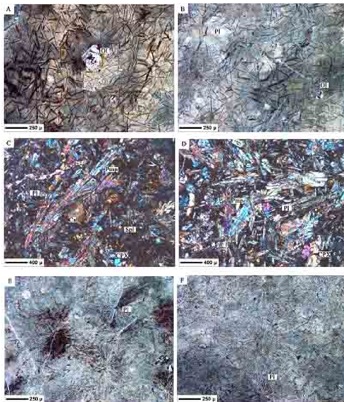
شکل ۴ تصاویر میکروسکوپیکی گدازه‌های بالشی افیولیت ملانژ ناین: (A) و (B): بازالت‌های الیون دار (ppl)، که شیشه‌های آن نیز دستخوش تبلور شده‌اند (دوتریفیکاسیون)؛ (C) و (D): بازالت‌های غنی از کلینوپیروکسن و پومپلئیت (xpl)، (E) و (F): بازالت‌های غنی از پلاژیوکلاز با بافت آبله-گون (ppl) (مخفف اسامی کانی‌ها برگرفته از [۱۹]). این تصاویر نتیجه، رخداد جدایش در ماگمای سازنده گدازه‌های بالشی هستند.
