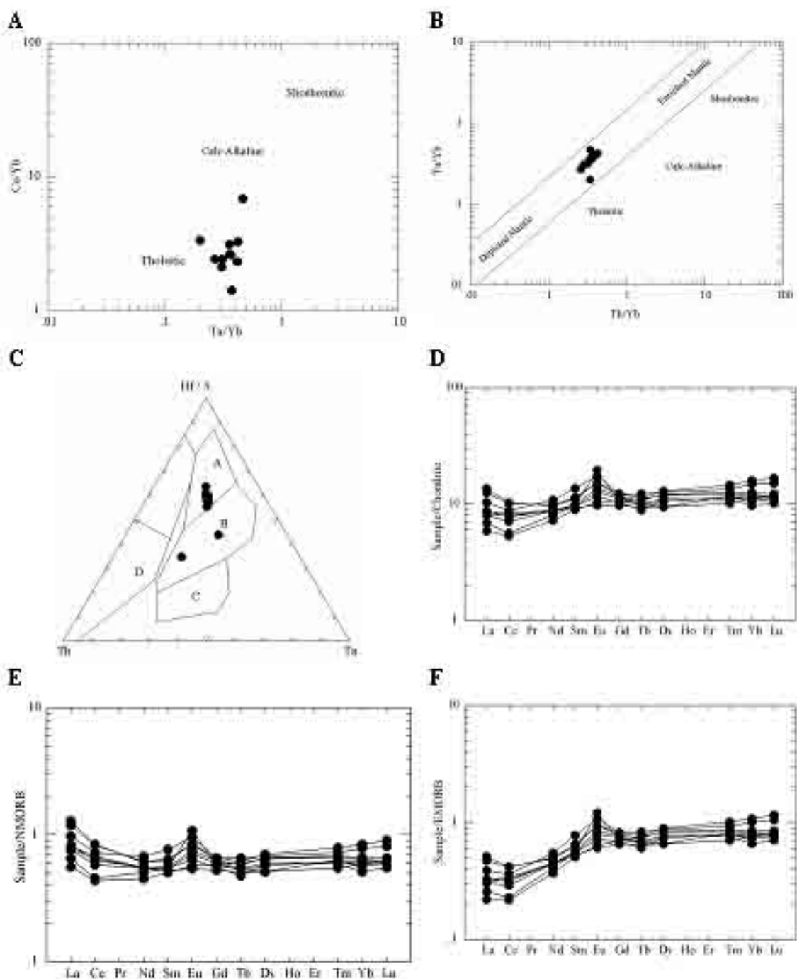
شکل ۷ (A) نمایش ترکیب سنگ کل گدازه‌های بالشی افیولیت ملائز نائین در نمودار Ce/Yb نسبت به Ta/Yb (برگرفته از [۲۴]); (B) نمایش ترکیب سنگ کل گدازه‌های بالشی افیولیت ملائز نائین در نمودار Ta/Yb نسبت به Th/Yb (برگرفته از [۲۴]); (C) نمایش ترکیب سنگ کل گدازه‌های بالشی افیولیت ملائز نائین در نمودار Th-Hf/3-Ta (برگرفته از [۲۵]); (D) نمودار بهنجارسازی عناصر نادر خاکی نسبت به کندریت؛ (E) نمودار بهنجارسازی عناصر نادر خاکی نسبت به NMORB؛ (F) نمودار بهنجارسازی عناصر نادر خاکی نسبت به EMORB.
