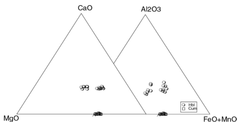
شکل ۴ ترکیب کانیه‌های آمفیبول فرومنیزین و آمفیبول کلسیک در نمودار ترکیبی \text{Mg}+\text{Ca}-(\text{Fe}+\text{Mn}) و \text{Mg}+\text{Al}_2\text{O}_3-(\text{Fe}+\text{Mn})
