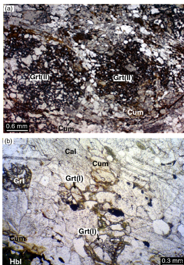
شکل ۲ (a) بافت پوئی کلیوبلاستیک در پورفیروبلاست گارنت. کانیهای کامینگتونیت، هورنبلند و کلسیت به صورت طویل شده برگرگی پیرامون پورفیروبلاست گارنت را تشکیل داده اند، PPL. (b) کانی های گارنت دانه ریز و بی شکل در زمینه گرانوبلاستیک، PPL.
