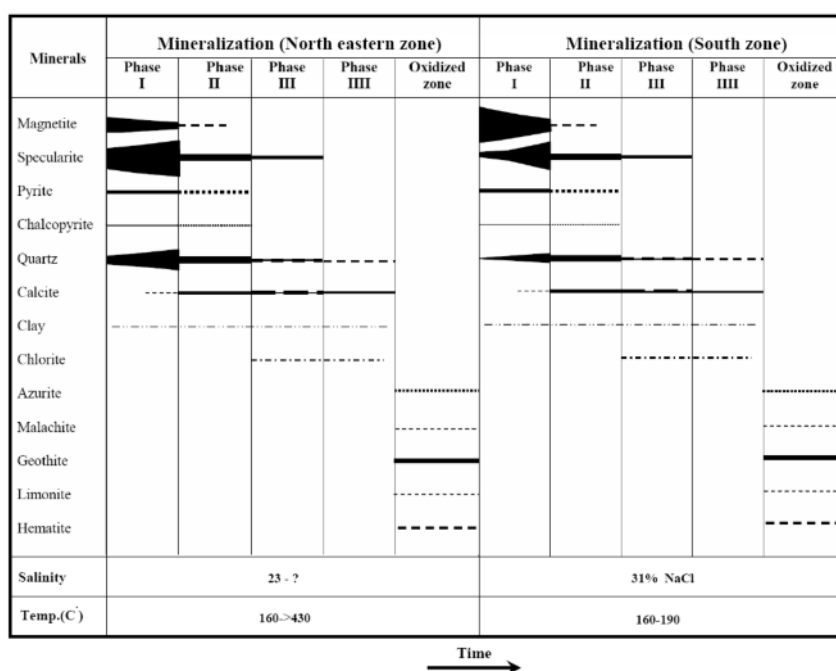
شکل ۴ دنباله پارائزی زونهای کانی‌سازی آهن.
