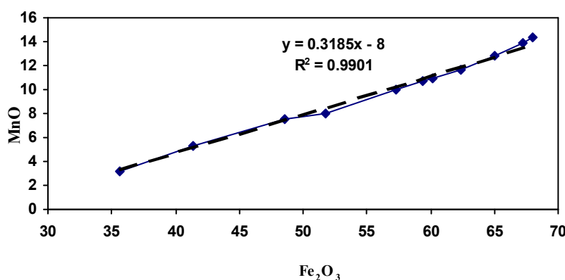
شکل ۱۰ نمودار MnO بر حسب Fe_2O_3
