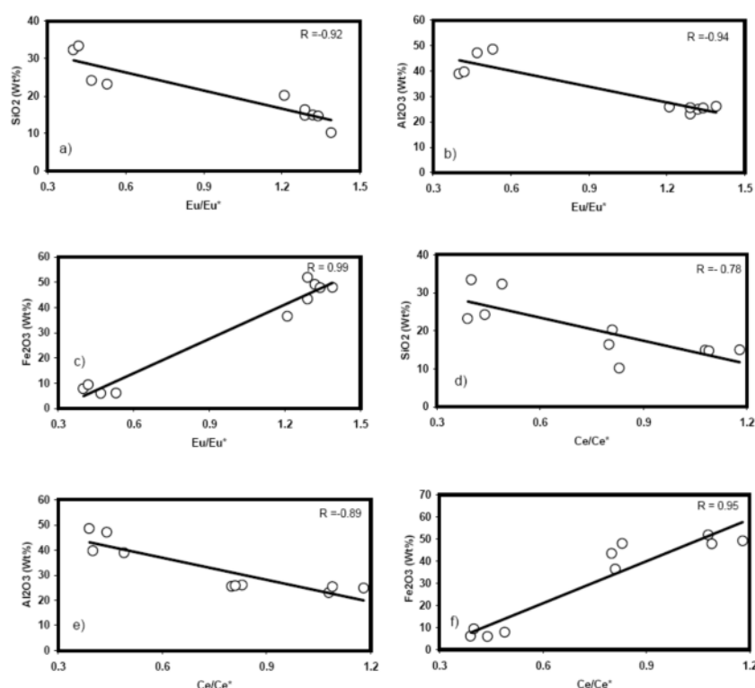
شکل ۷ نمودارهای تغییرات بیهنجاری Eu در برابر SiO 2 (a)، Al 2 O 3 (b)، Fe 2 O 3 (c) و بی هنجاری Ce در برابر SiO 2 (d)، Al 2 O 3 (e) و Fe 2 O 3 (f) در طی فرایندهای بوکسیتی شدن در شمال خاوری بوکان.
