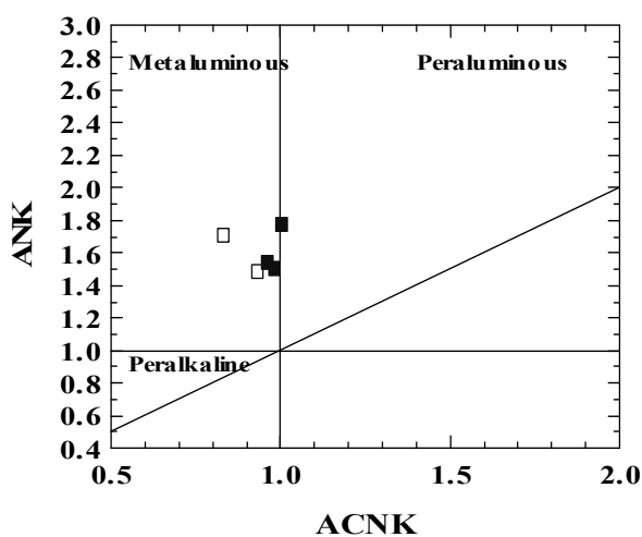
شکل ۵ تعیین میزان آلومینه گرانیت چاه ترش [۱].
