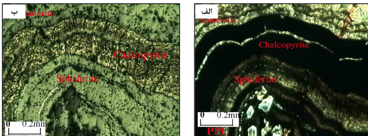
شکل ۷ بافت کلوفر (ریتمیک) از کانی اسفالریت در نور PPL عبوری در الف و نور بازتابی در ب.
