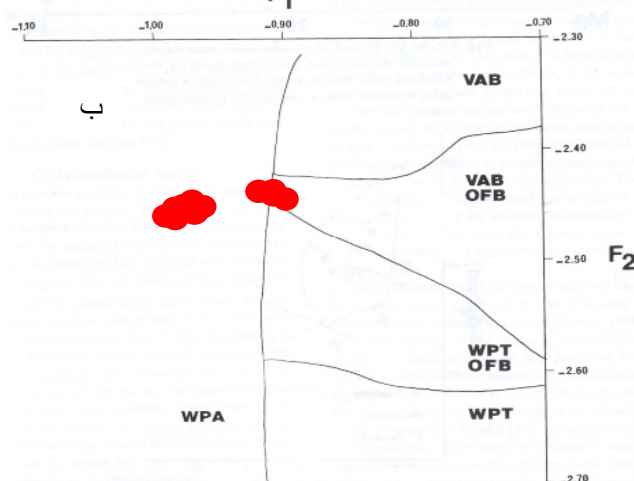
شکل ۹ الف نمودار \text{SiO}_2/\text{Al}_2\text{O}_3 [۱۷] و جایگاه پیروکسنهای سازند هرمز روی آن، ب نمودار F_1 - F_2 و موقعیت کلینوپیروکسنهای ماگمایی سازند هرمز روی آن [۱۹]
