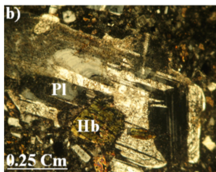
شکل ۳ تصاویر میکروسکوپی از سنگ های آتشفشانی منطقه. (a) پلاژیوکلاز (Pl) در حال سریسیستی شدن، (b) منطقه بندی نوسانی در پلاژیوکلاز و همراهی با هورنبلند (Hb).
