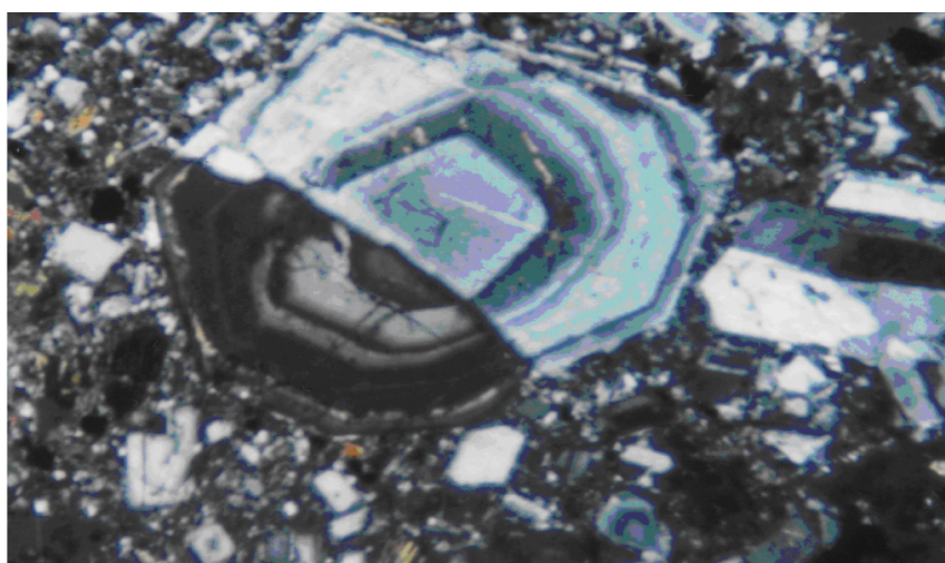
شکل ۲ پدیده (منطقه‌بندی) در پلاژیوکلازهای موجود در کوارتز دیوریت‌های منطقه.
