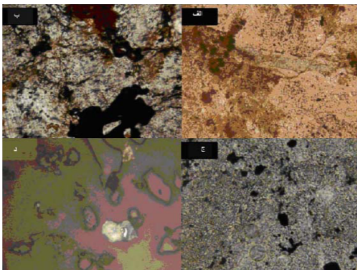
شکل ۶ الف) (مالاکیت) به صورت پرشدگی در فضای خالی و گوتیت ناشی از پیریت در زمینه سیلیسی. ب) کانی‌های کدر (مگنتیت) و نیمه شفاف و بافت داربستی ج) کانی‌های کدر (مگنتیت) در اندازه‌های مختلف با بافت پراکنده (زمینه دگرسان شده است). د) کالکوپیریت، دیژنیت و پیریت باقی مانده به صورت درگیر.
