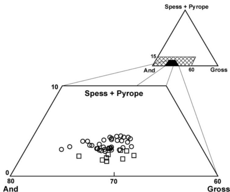
شکل ۴ ترکیب گارنت‌های مورد بررسی در نمودار And - Gross - (Spess + Pyrope)؛ گستره گارنت‌های غنی از Ti با هاشور مشخص شده است [۱۷].
