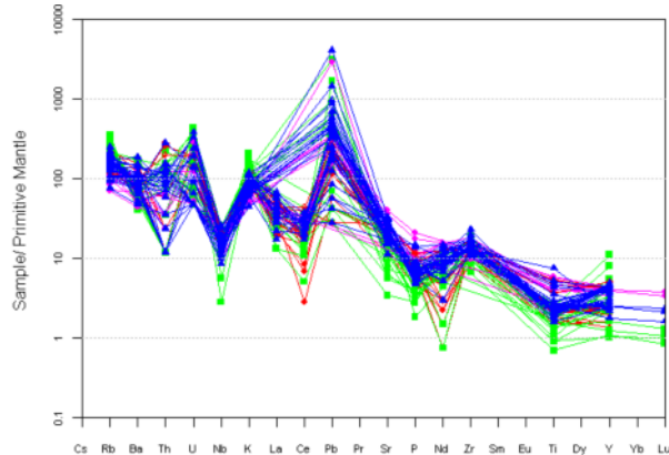
ب - نمودار چند عنصری بهنجار شده به گوشتهٔ اولیه [۳۹] تمامی گروه‌های سنگ‌های نفوذی منطقهٔ زاهدان. شکل ۱۲ نمودارهای عناصر خاکی کمیاب و چند عنصری بهنجار شده به کندریت و گوشته اولیه برای سنگ‌های آذرین منطقهٔ زاهدان.
