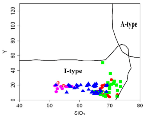
ج - نمودار تغییرات \text{SiO}_2 نسبت به Y [۵۸].
