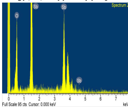
شکل ۳ نمودار EDX نانوذرات اکسید آنتیموان
