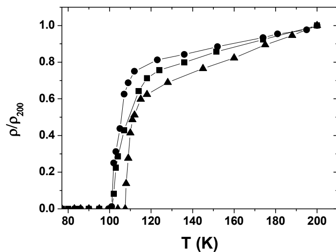
شکل ۵ نمودارهای \rho - T برحسب مقادیر متفاوت نانوذرات اکسید آنتیموان x = 0.0 (■)، x = 0.5 (▲) و x = 0.7 (●) با زمان پخت ۲۷۰ ساعت.
