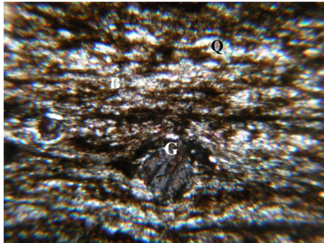
شکل ۳ جهت یافتگی کانی‌های برگه‌ای میکا (xpl, \times 100 ): Q: کوارتز - B: بیوتیت - G: گارنت.
