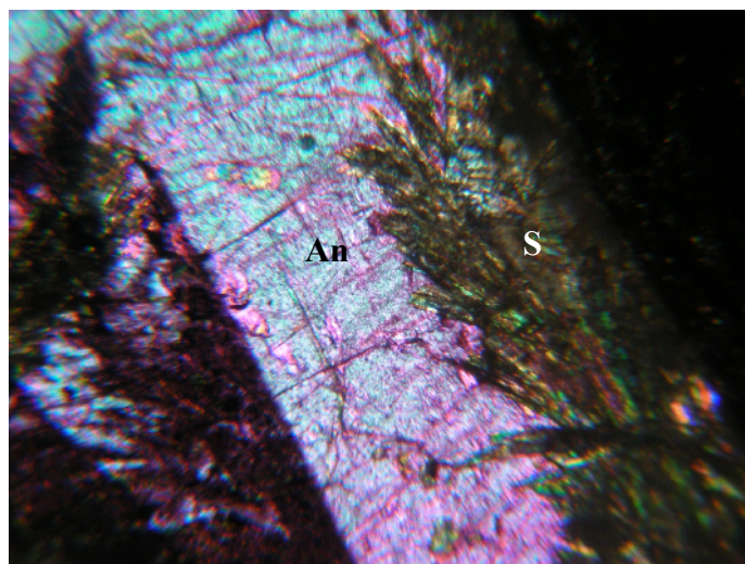
شکل ۵ آندالوزیت در حال تبدیل به سیلیمانیت (An (xpl, \times 100 ): آندالوزیت - S: سیلیمانیت.
