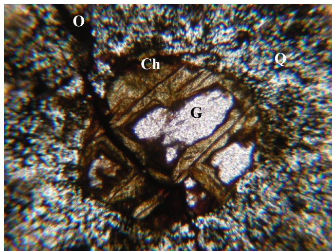
شکل ۴ گارنت در حال تجزیه به کلریت (ppl, \times 100 ): Q: کوارتز - Ch: کلریت - G: گارنت - O: کانی‌های کدر.
