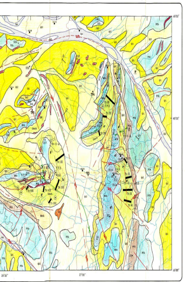
شکل ۲ نقشه‌ی زمین‌شناسی منطقه‌ی مورد بررسی آندالوزیت میشدوان بافق [۶].
