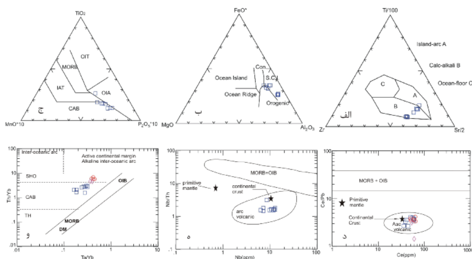
شکل ۹ تعیین محیط زمین‌ساختی سنگ‌های آتشفشانی منطقه‌ی مورد بررسی با استفاده از نمودارهای، (الف) [۲۲]، (ب) [۲۳]، (ج) [۲۴]، (د) [۲۵]، (ه) [۲۶، ۲۴]، (و) [۲۷] (□) پیروکسن‌بازالت، تراکی‌بازالت و تراکی‌آندزیت، ◇ آندزیت، ○ ریولیت و تراکی‌داسیت.
