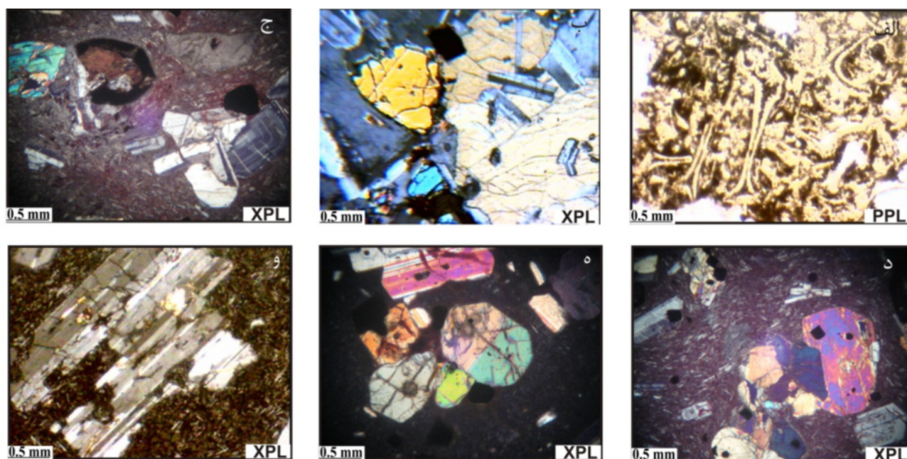
شکل ۴ تصاویر میکروسکوپی از: (الف) شاردهای شیشه‌ای فراوان با اشکال مختلف در ریولیت. (ب) بافت افیتیک (وجود نفوذی‌های پلاژیوکلاز، کدر و کلینوپیروکسن در فنوکریست‌های پیروکسن) در بازالت (ج) فنوکریست‌های آمفیبول با حاشیه‌ی سوخته (اپاسیتی شده) و پلاژیوکلاز دارای زونینگ در زمینه‌ای متشکل از میکروولیت‌های پلاژیوکلاز با بافت نمدی در تراکی‌آندزیت. (د) بافت گلومروپرفیری و غربالی در بلور پلاژیوکلاز در زمینه‌ای متشکل از میکروولیت‌های پلاژیوکلاز با بافت جریانی در تراکی‌آندزیت. (ه) بلورهای اتومورف کلینوپیروکسن با ماکل تیغه‌ای در یک زمینه-ی شیشه‌ای در آندزیت. (و) آثار خوردگی در بلور پلاژیوکلاز در آندزیت.
