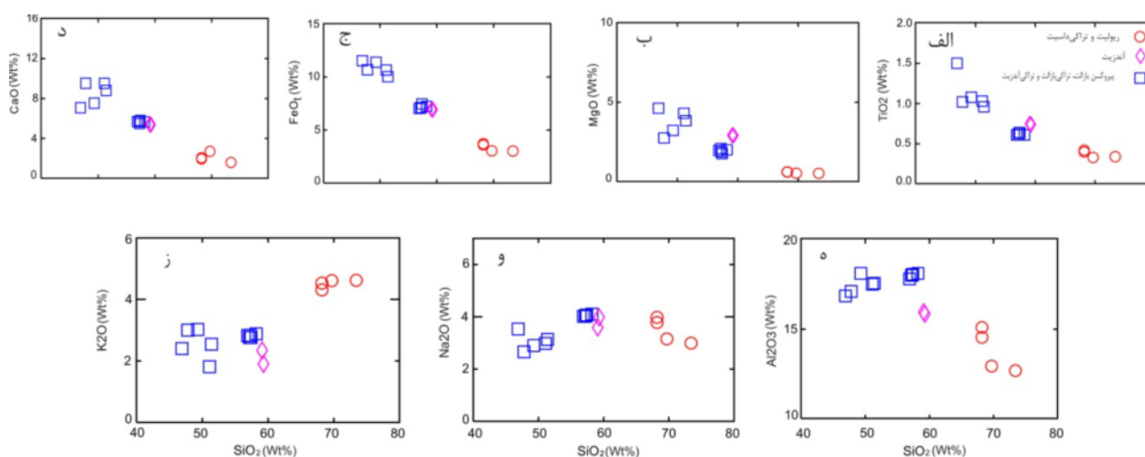
شکل ۵ تغییرات اکسیدهای اصلی نسبت به \text{SiO}_2 در سنگ‌های آتشفشانی منطقه‌ی مورد بررسی.
