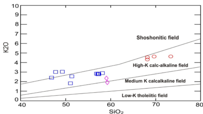
شکل ۸ نمونه‌های منطقه روی نمودار دوتایی K_2O نسبت به SiO_2 [۲۱]. معرف ماهیت آهکی و قلیایی با پتاسیم بالا تا شوشونیتی سنگ‌های منطقه است. (□) پیروکسن‌بازالت، تراکی‌بازالت و تراکی‌آندزیت، (◇) آندزیت، (○) ریولیت و تراکی‌داسیت.
