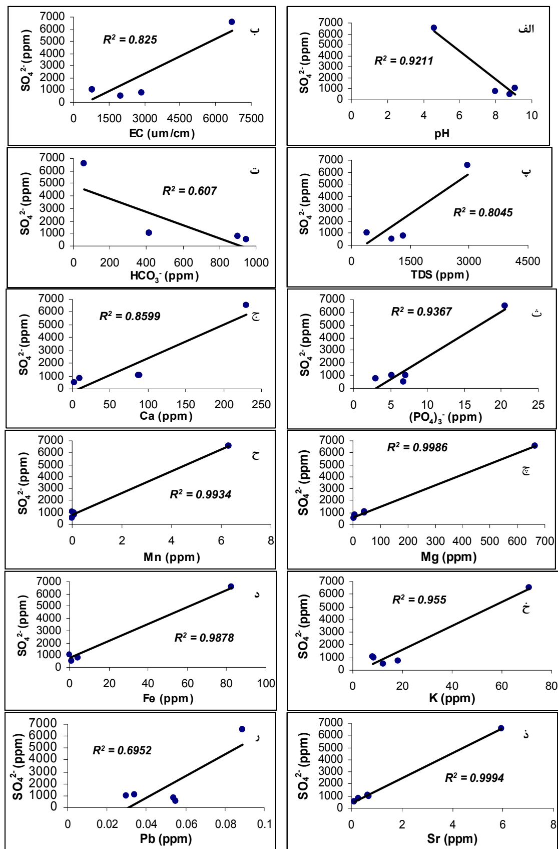
شکل ۳ نمودار پراکنش \text{SO}_4^{2-} در مقابل الف pH، ب EC، پ TDS، ت \text{HCO}_3^- ، ث (\text{PO}_4)_3^- ، ج Ca، چ Mg، ح Mn، د Fe، ز Sr، ر Pb.
