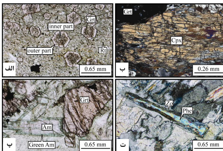
شکل ۳ تصاویر میکروسکوپی از اکلوزیت‌های شاندرمن، الف) نمایش بخش مرکزی و خارجی گارنت‌ها (PPL) ب) کلینوپیروکسن و گارنت‌های اوج دگرگونی (XPL) پ) آمفیبول‌های منطقه‌ای و شکستگی‌های موازی در گارنت (PPL) ت) رشد تأخیری زوئیزیت در اطراف فنزیت (XPL). علائم اختصاری کانی‌ها از [۱۴]: گارنت: Grt، روتیل: Rt، کلینوپیروکسن: Cpx، آمفیبول: Am، زوئیزیت: Zo، فنزیت: Phe.
