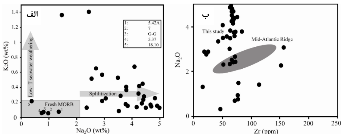
شکل ۶ الف) نمودار Na 2 O نسبت به K 2 O، بیشتر نمونه‌ها روند اسپیلیتی شدن را نشان می‌دهند [۲۳] و ب) نمودار Zr نسبت به Na 2 O و نمایش پراکندگی داده‌ها (برای توضیحات بیشتر به متن مراجعه شود).
