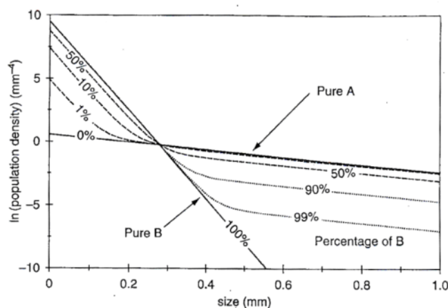
شکل ۳ اضافه شدن دو CSD خطی به یکدیگر و ایجاد CSD منحنی وار. شیب‌های اولیه دو تشکیل دهنده‌ی CSD برای اندازه‌های بزرگ و کوچک حفظ می‌شود ولی عرض از مبدا آن‌ها حفظ نمی‌شود.
