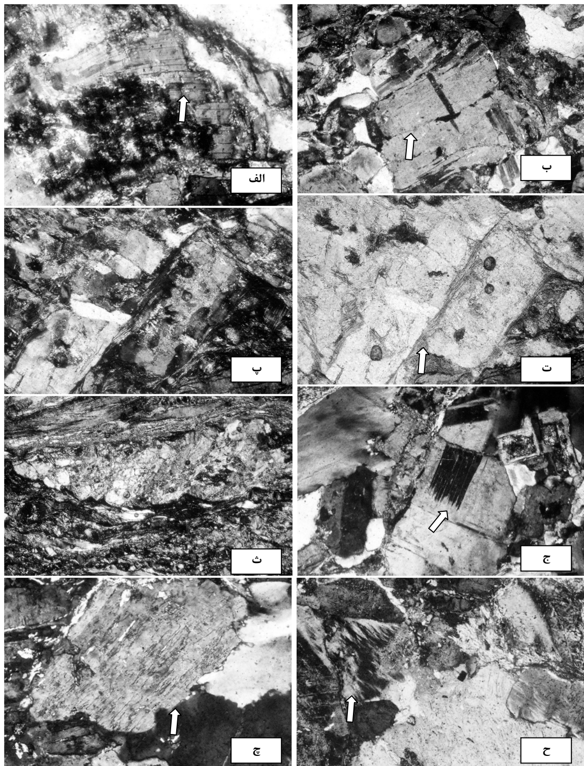
شکل ۶ تصاویر میکروسکوپی از ریز ساختارها در فلدسپات‌ها در زون‌های برشی مورد بررسی در نور XPL (طول تصاویر برابر ۱/۲ میلی‌متر است). (الف) خمیدگی ماکل‌ها در پلاژیوکلازها. (ب) گسترش شکستگی‌ها، سطوح لغزش در فلدسپات‌ها (آلبیت). (پ) ساختار بودین‌های دومینویی در پلاژیوکلازها در نور XPL و (ت) در نور PPL. (ث) ریز ساختار دو مینویی در پلاژیوکلاز. این ساختار معرف سمت و سوی برش راستگرد در زون-های برشی مورد بررسی است. (ج) ماکل‌های تغییر ساختاری در پلاژیوکلازها. (چ) حاشیه لخته‌ای (lobate) میان کوارتز و فلدسپات. (ح) پرتیت‌های شعله‌ای در فلدسپات‌های قلیایی.
