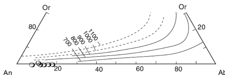
شکل ۸. تعیین دمای دو فلدسپار در نمونه گابروئی AZ17 از روش دماسنجی دو فلدسپار [۲۴] برای فرایند یاد شده دما بین ۷۰۰-۸۰۰ درجه سانتی گراد ارزیابی می شود.
