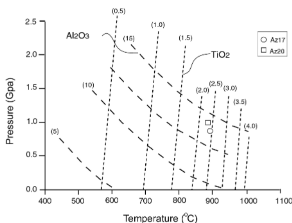
شکل ۹. دما-فشارسنجی با تک کانی آمفیبول بر اساس مقدار اکسیدهای آلومینیوم و تیتانیم در این کانی [۲۵]. فشار در حدود ۹-۱۱ کیلو بار و دما نزدیک به ۹۰۰ درجه سانتی گراد برای تبلور آمفیبول های منطقه ارزیابی می شود. فشار تبلور آمفیبول های موجود در سنگ های اولترامافیک در حدود ۲ کیلو بار بالاتر از فشار تشکیل گابروهاست.
