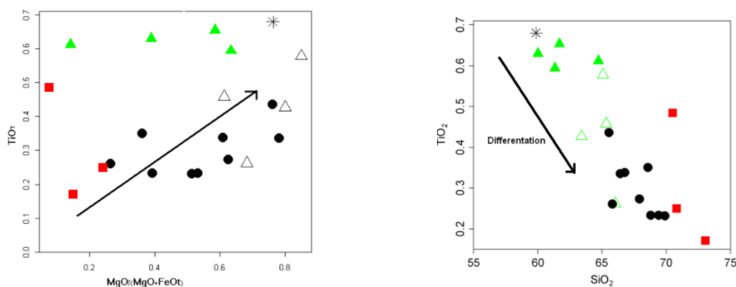
شکل ۹ نمودار \text{TiO}_2\text{-MgO}/(\text{MgO} + \text{FeOt}) از [۱۸] و نمودار \text{TiO}_2\text{-SiO}_2 از [۱۹] برای نمایش روندهای وابسته به پدیده‌های تبلور جدایشی طی تشکیل سنگ‌های آذرین منطقه‌ی مشکان.
