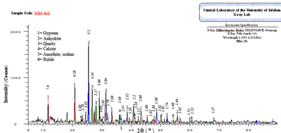
شکل ۱۹ نمودار XRD نمونه سفید.
