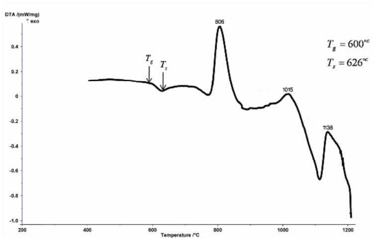
شکل ۶ نمودار DTA نمونه M_3 با سرعت گرمادهی 10^{\circ}\text{C/min}
