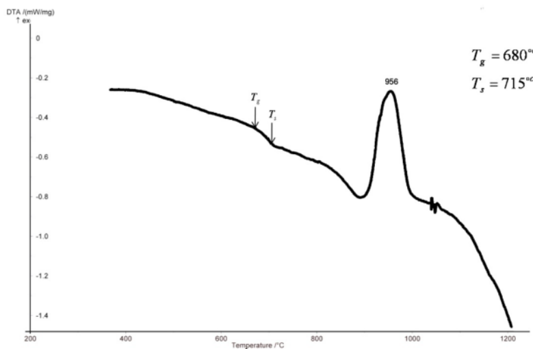
شکل ۵ نمودار DTA نمونه M_2 با سرعت گرمادهی 10^{\circ}\text{C/min}
