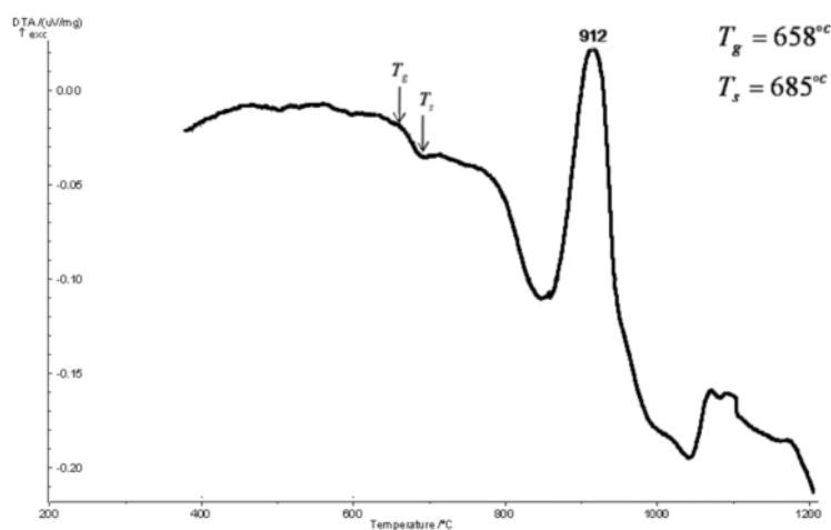
شکل ۴ نمودار DTA نمونه M_1 با سرعت گرمادهی 10^{\circ}\text{C/min}
