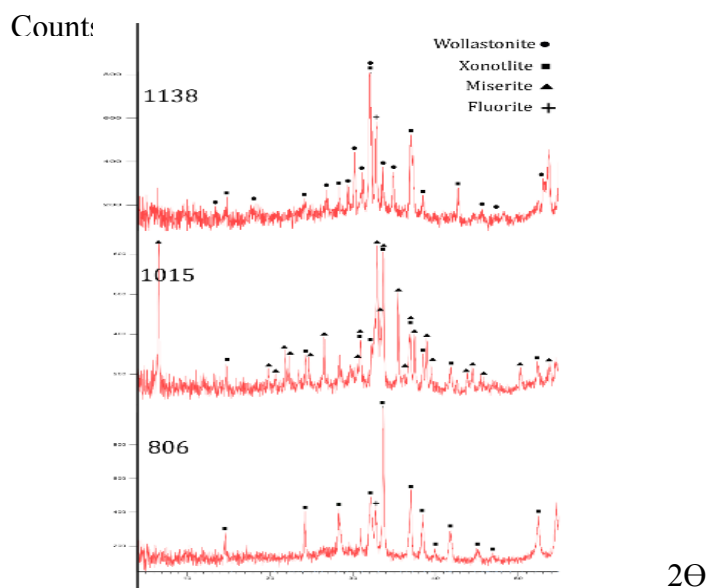
شکل ۹ نمودار پراش پرتو ایکس نمونه M_3 در دماهای 806^\circ C ، 1015^\circ C و 1138^\circ C
