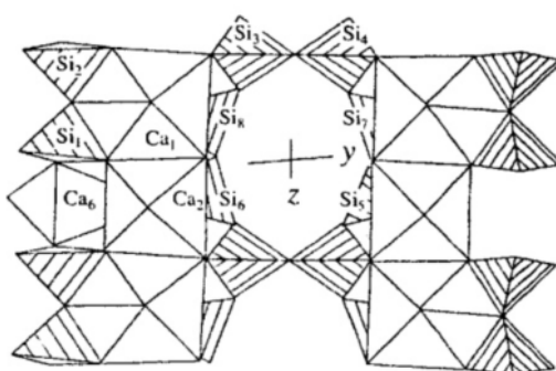
شکل ۳ موقعیت رادیکال‌های سیلیکاتی [Si_{11}O_3]^{12-} و دی‌ارتوگروه‌های [Si_2O_7]^{6-} در ساختار میسریت [۹].
