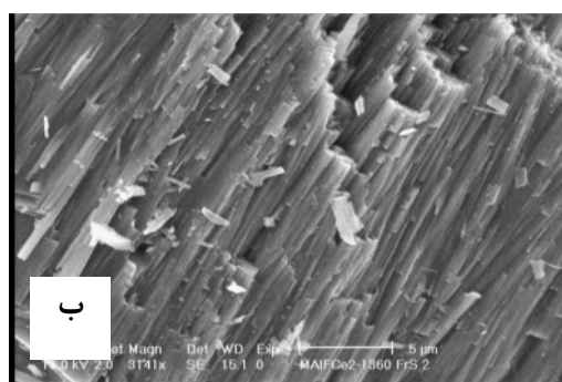
شکل ۱۰ تصویر SEM از نمونه M_3 در دمای 1015^\circ C با دو بزرگنمایی مختلف.
