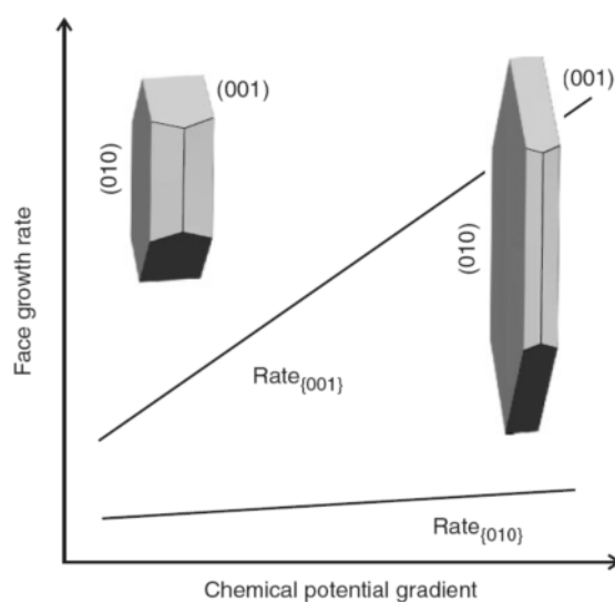
شکل ۸ واکنش احتمالی سرعت‌های رشد وجوه پلاژیوکلاز به تغییرات پتانسیل شیمیایی پیرامون بلور در حال رشد [۲۰]. سطح (۰۰۱) به‌عنوان سطح حاشیه‌ی تخته انتخاب شده است (فرض بر این است که سرعت رشد سطوح (۱۱۰)، (۱۰۱) و (۱۱۰) معادل با سطح (۰۰۱) است). اندازه‌ی کلی بلور نمایش داده شده سرعت رشد و زمان تبلور را بازتاب می‌دهد.
