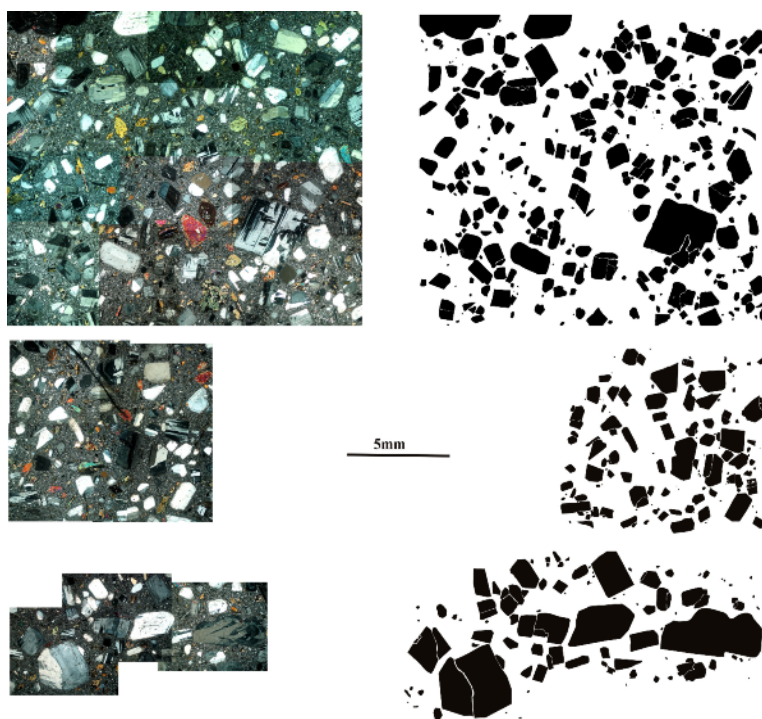
شکل ۲ تصاویر چند ناحیه از مقطع MAD4 (سمت چپ) و تصاویر پردازش شده پس از رسم محیط بلورهای پلاژیوکلاز (سمت راست). مقیاس همه‌ی تصاویر یکسان است. در تهیه و پردازش تصاویر بالا از تلفیق ۲۳ عکس دیجیتالی استفاده شده است.
