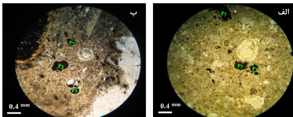
شکل ۲ مقاطع نازک پیریت اتوژنیک در رسوب‌های دریایی گودال نانکای. الف) پیریت اتوژنیک به مقدار کم در زمینه‌ی رسوب‌ها. ب) پیریت اتوژنیک در حجره‌های فرامینفرا.
