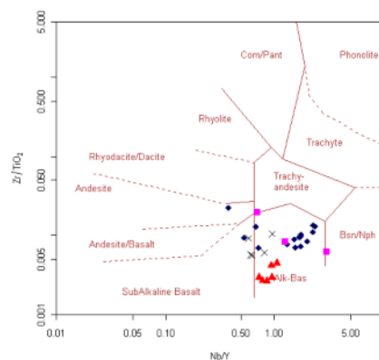
شکل ۱۲ موقعیت نمونه‌های مورد بررسی در نمودار Zr/TiO_2 -Nb/Y [۱۶] (ایبانه ◆، دالمه ■، زفره ▲، انارک (پل خاوند) ×).
