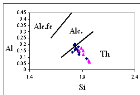
شکل ۸ تصویر ترکیب کلینوپیروکسن‌های مورد بررسی در نمودار \text{Al}/\text{Si} [۱۲] Alkaline feldspathoids (Alc.fe), Th: Tholeiite, Alc: Alkaline (ایبانه ♦، پل خاوند ▲)
