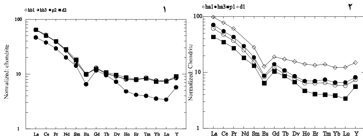
شکل ۷ الف) ۱ و ۲) نمودار عناصر نادر خاکی بهنجار شده نسبت به کندریت در دو نیمرخ مورد بررسی، بیانگر شیب نزولی، تهی شدگی در یوروپیم و کاهش غلظت از LREEs به طرف HREEs.
