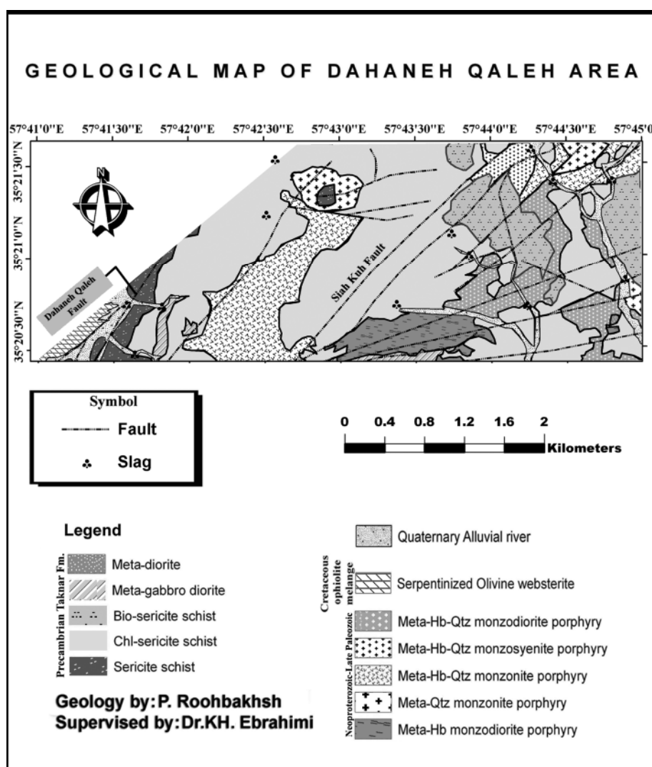
شکل ۳ نقشه زمین‌شناسی گستره‌ی پی‌جویی دهن قلعہ.
