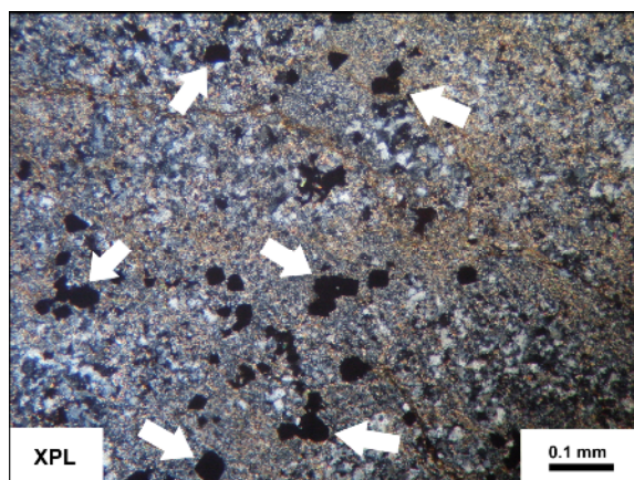
شکل ۱۴ نمایی از پیریت‌های پراکنده در متن سرسپت شیست‌های محدوده دهن قلع.
