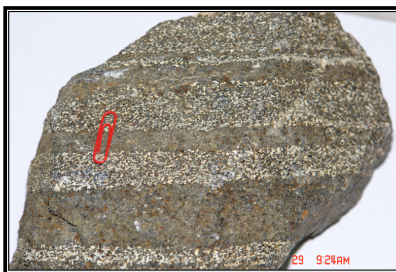
شکل ۶. لایه‌بندی مودال تناوبی در گابروی لایه‌ای گروه دوم با تناوبی از اولیوین گابرو و اولیوین کلینوپیروکسنیت پلاژیوکلازدار.
