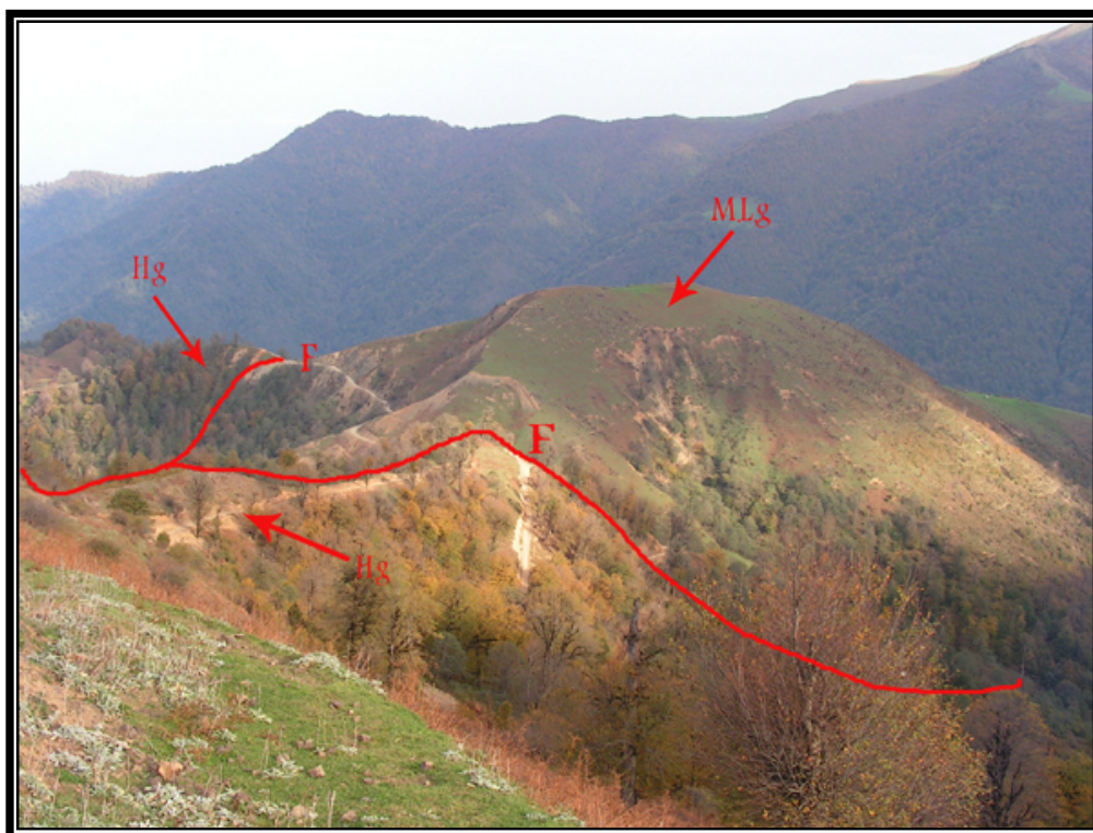
شکل ۵. برونزد گابروی لایه‌ای گروه دوم (M.L.g) که با همبندی گسله با واحد گابروهای غیر لایه‌ای گروه اول (H.g) دیده می‌شود. (دید به سمت شمال شرق)
