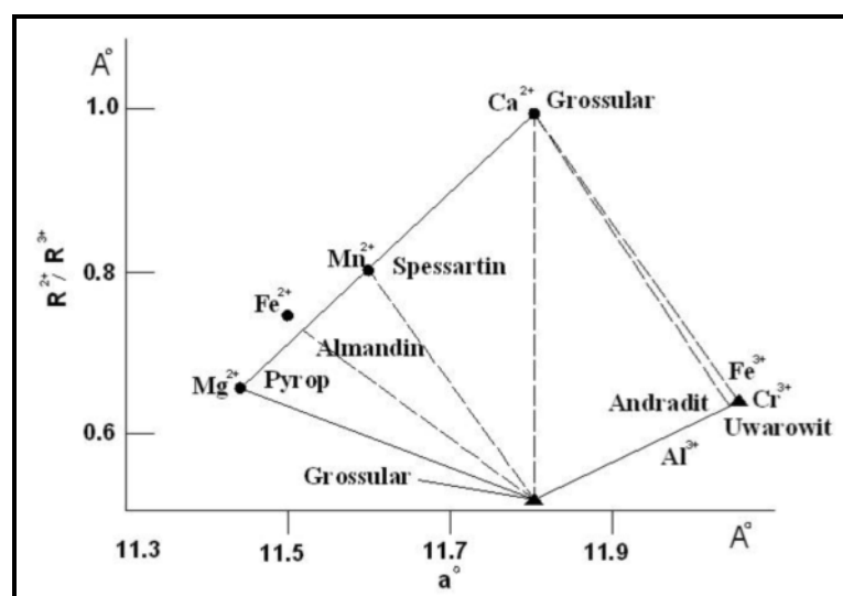
شکل ۱۱ تغییر ترکیب شیمیایی بلورهای گارنت وابسته به نسبت کاتیون‌های دو ظرفیتی به سه ظرفیتی و اندازه‌ی یاخته‌ی یک [۹].
