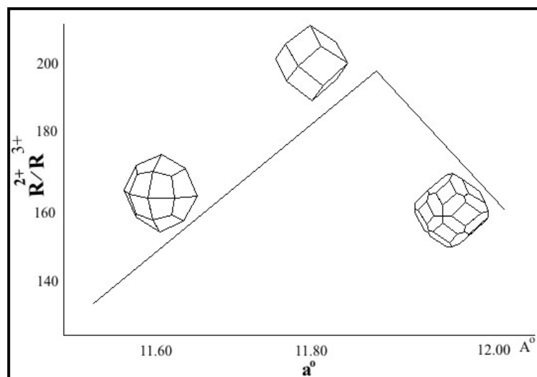
شکل ۱۰ تغییر پیکربندی بلورهای گارنت وابسته به نسبت کاتیون‌های دو ظرفیتی به سه ظرفیتی و اندازه‌ی یاخته‌ی یک [۸].
