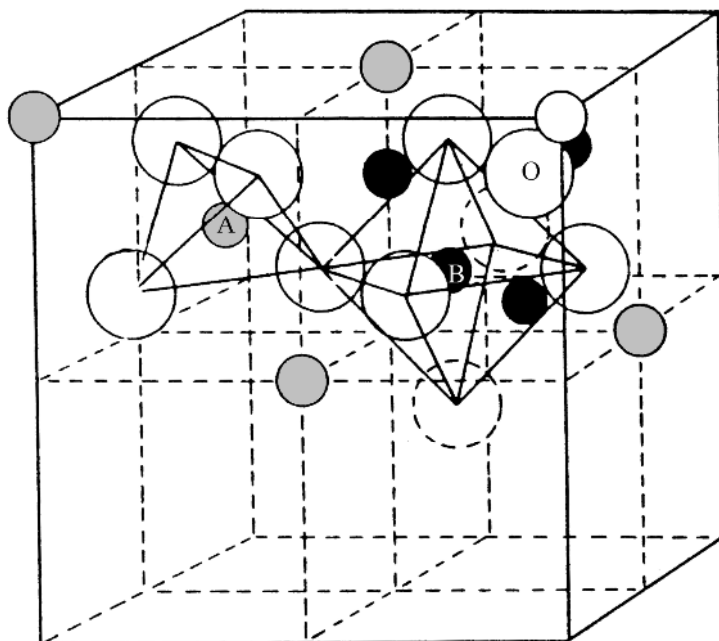
شکل ۱ ساختار بلوری اسپینل با فرمول AB_2O_4 . کره‌های سفید بزرگ یون‌های اکسیژن و کره‌های خاکستری و سیاه کوچک به ترتیب نشان دهنده جایگاه‌های چهار وجهی (A) و هشت وجهی (B).
