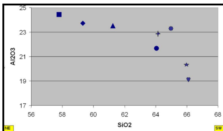
شکل ۵. تغییرات میزان آلومینا نسبت به میزان سیلیس.
