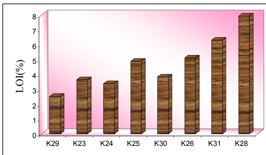
شکل ۶ مقادیر LOI به نمونه‌های شیخ آباد.
