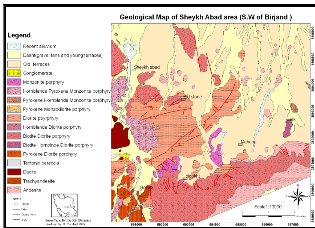
شکل ۲ نقشه ۱:۱۰۰۰۰ زمین‌شناسی منطقه‌ی شیخ آباد [۸].
