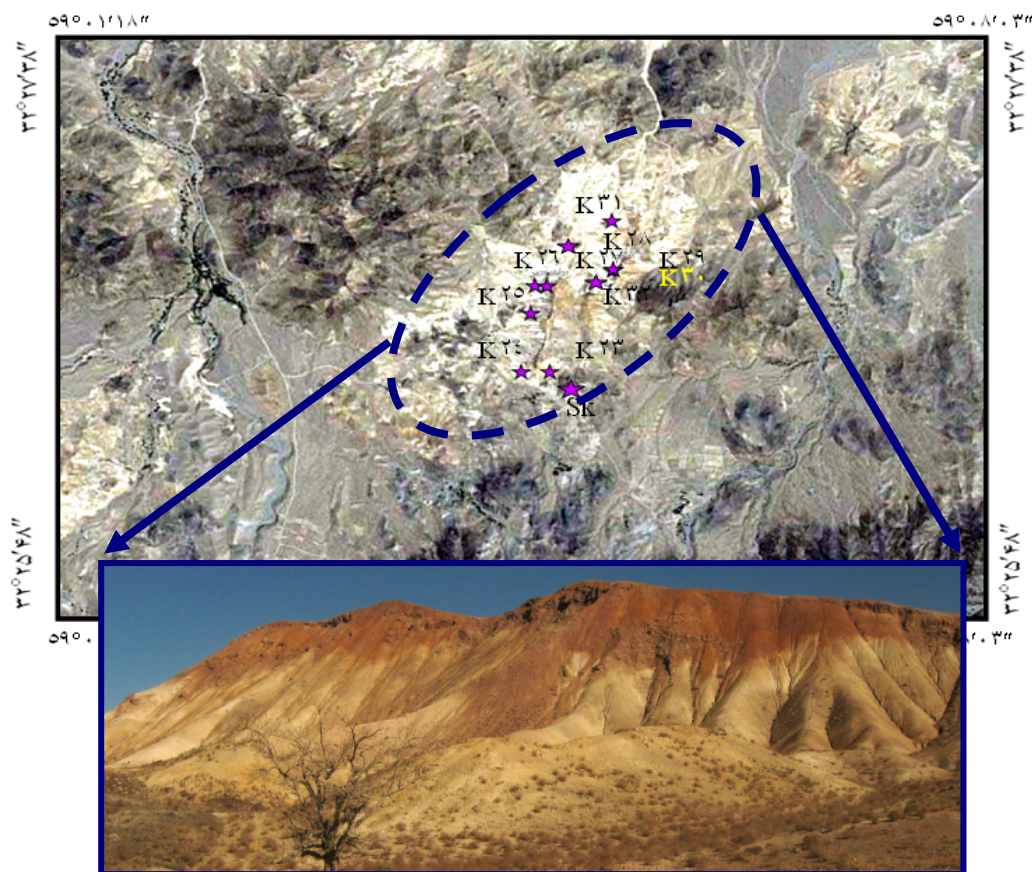
شکل ۳ تصویر ماهواره‌ای از آرژلیک دگرسان منطقه‌ی شیخ آباد و موقعیت نمونه‌های کائولینیتی برداشت شده
