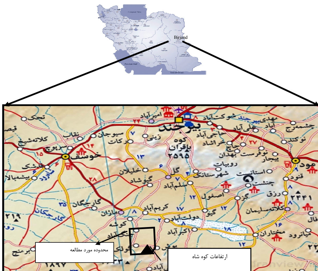
شکل ۱ موقعیت منطقه‌ی شیخ آباد [۷].
