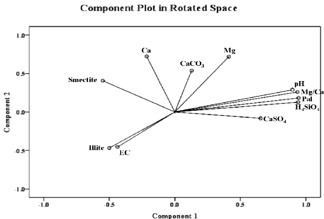
شکل ۷ نمایش تحلیل فاکتورها به روش تجزیه‌ی مولفه‌های اصلی که بیانگر ارتباط بین پالیگورسکیت و متغیرهای دیگر در مواد مادری و خاک-های مورد بررسی است.
