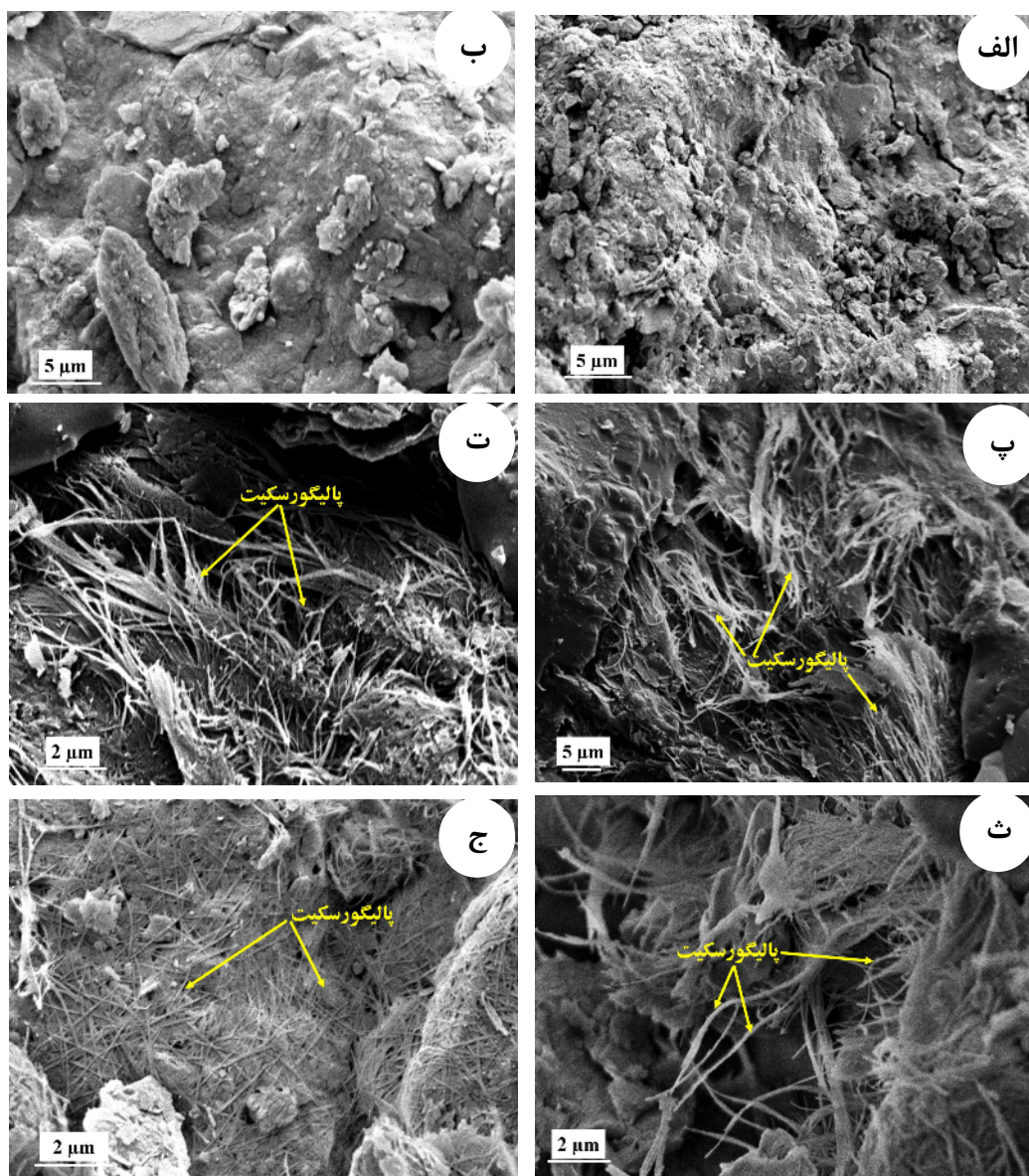
شکل ۴ ریز نگاشت میکروسکوپ الکترونی روبشی در مواد مادری با سن ترشیری. تصاویر "الف" و "ب" بیانگر عدم حضور کانی پالیکورسکیت به ترتیب در رسوب‌های ائوسن و الیگوسن (مواد مادری نیمرخ‌های ۱ و ۲) و تصاویر "پ تا ج" نیز حضور این کانی را به ترتیب در رسوب‌های الیگوسن - میوسن، میوسن و پلیوسن (مواد مادری نیمرخ‌های ۳، ۴، ۵ و ۶) در منطقه‌ی مورد بررسی نشان می‌دهند.
