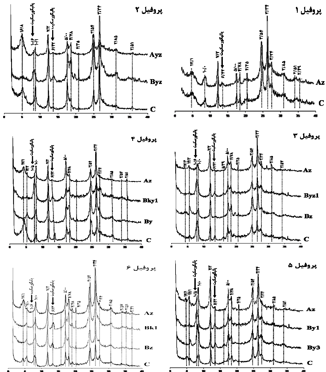
شکل ۳ پراش نگاشت‌های پرتو ایکس تیمار "منیزیوم اشباع + اتیلن گلیکول" در بخش رس خاک‌ها و مواد مادری مورد بررسی که نمایانگر فراوانی بیشتر پالیگورسکیت (قله اختصاصی ۶/۴۲ آنگستروم) در افق‌های انباشت گچ (By) در مقایسه با افق‌های انباشت نمک (Az و Bz) می‌باشند. اعداد قله‌ها بر حسب آنگستروم ارائه شده‌اند.
