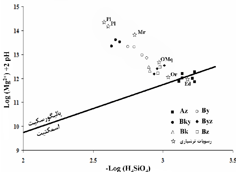
شکل ۸. نمودار پایداری سیستم پالیکورسکیت- اسمکتیت بر اساس ترکیب شیمیایی نمونه‌های خاک و مواد مادری مورد بررسی که بیانگر پایداری بیشتر پالیکورسکیت در افق‌های انباشت گچ نسبت به افق‌های انباشت آهک و نمک، و ناپایداری نسبی این کانی در برخی افق‌های سطحی و رسوب‌های اتوسن است.
