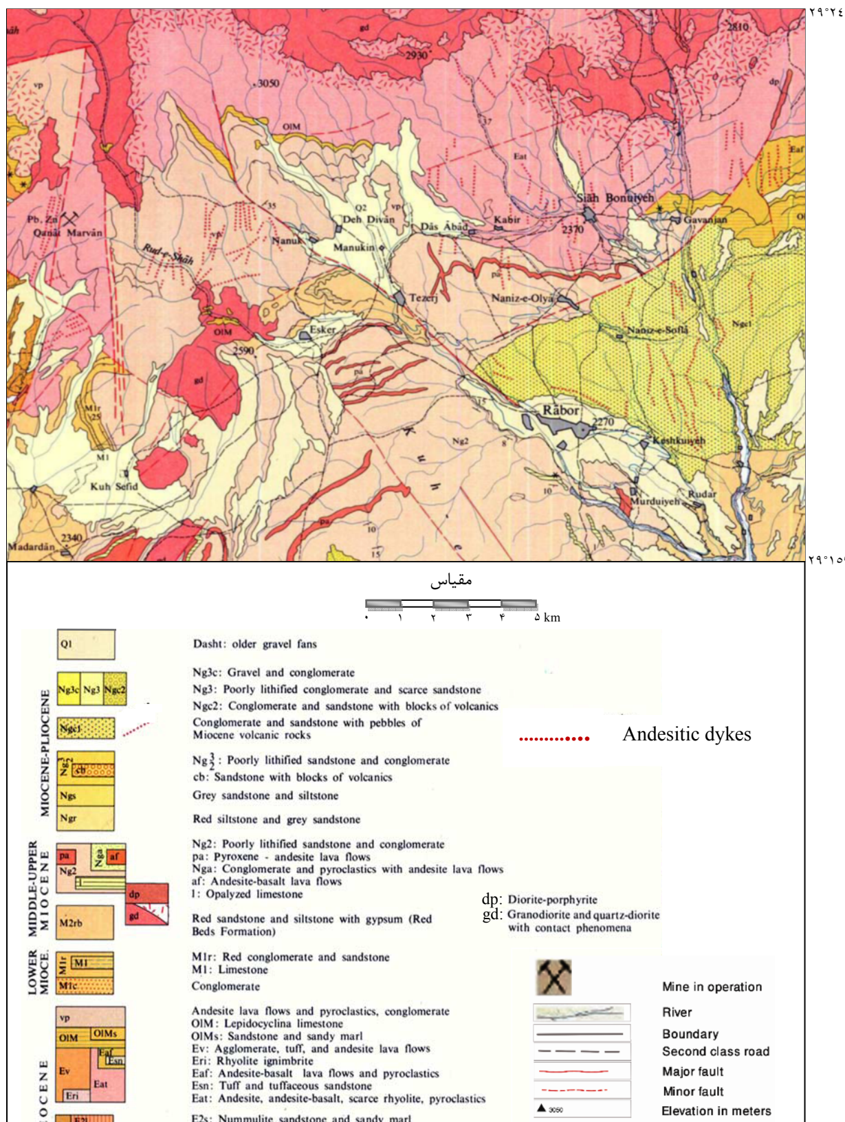
شکل ۲ نقشه‌ی زمین‌شناسی منطقه‌ی مورد بررسی (اقتباس از نقشه‌ی ۱:۱۰۰۰۰۰ بافت، سازمان زمین‌شناسی و اکتشافات معدنی کشور ۱۳۳۸).
