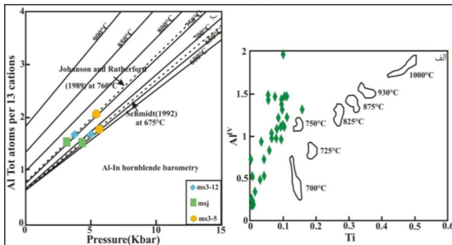
شکل ۸ الف: محاسبه دمای تشکیل آمفیبول‌های نمونه‌های مورد بررسی براساس روش هلز [۲۸]، ب: فشار (کیلو بار) نسبت به Al^T رسم شده است [۱۷، ۱۵] می‌توان گستره دمایی بین ۶۰۰-۷۵۰°C را برای منیزیهورنبلندهای مورد بررسی برآورد کرد.
