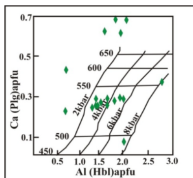
شکل ۱۰ دما-فشار، سنج هورنلند-یلاژ یوکلار: برای تعیین گستره‌ی دما-فشار، آمفیبولیت‌ها برگرفته از [۳۲].
