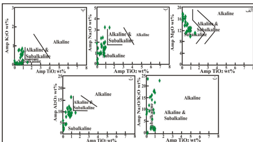
شکل ۳ در نمودارهای \text{TiO}_2 نسبت به (الف) \text{MgO} ، (ب) \text{Na}_2\text{O} ، (پ) \text{K}_2\text{O} ، (ت) \text{Na}_2\text{O}/\text{K}_2\text{O} و (ث) \text{Al}_2\text{O}_3 حاصل از آنالیز آمفیبول‌ها ماهیت ماگما به نیمه‌قلیایی تمایل دارد [۹].
