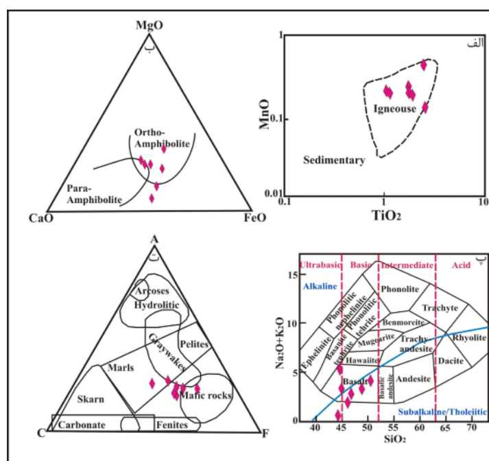
شکل ۱۲ الف: براساس نمودار [۳۶]، پروتولیت آمفیبولیت‌های منطقه آذرین است، ب: نمودار مثلثی MgO-CaO-FeO برای جدایی پارامفیبولیت و ارتوآمفیبولیت [۳۷]، پ: نمودار مجموع قلیایی-سیلیس [۳۸] که نمونه‌های مورد بررسی در این نمودار در گسترده‌ی بازالت قرار گرفته‌اند، ت: تعیین نوع سنگ مادر رسوبی نمونه‌های مورد مطالعه با استفاده از نمودار سه تایی ACF، [۳۹، ۴۰] F = \text{MgO} + \text{MnO} + \text{FeO} و A = (\text{Al}_2\text{O}_3) + (\text{Fe}_2\text{O}_3) - (\text{Na}_2\text{O} + \text{K}_2\text{O}) ، C = \text{CaO} - 3.3 \text{ P}_2\text{O}_5
