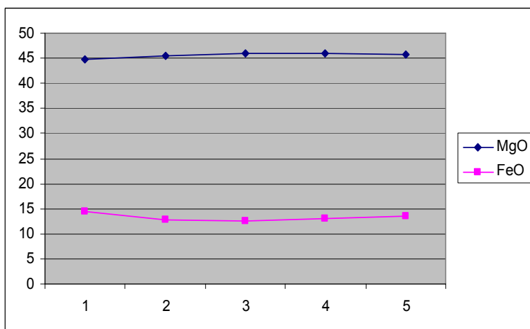
شکل ۱۲ نوسان‌های آهن و منیزیم در بلور الیوین نشان داده شده در نمونه‌ی بازالتی شکل ۱۱.
