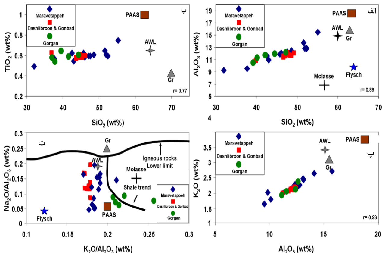
شکل ۳ نمودارهای (الف): Al_2O_3 نسبت به SiO_2 ، (ب): TiO_2 نسبت به SiO_2 ، (پ): K_2O نسبت به Al_2O_3 و (ت): Na_2O/Al_2O_3 نسبت به K_2O/Al_2O_3 در مقایسه با ترکیب میانگین جهانی بادرقتا (AWL) [۳۰]، شیل رسوبی میانگین پسا آرکئن استرالیا (PAAS) [۲۳]، ماسه سنگ مولاسی (Molasse) [۲۵]، گرانیت شاهد کارپاتیانس (Carpathians Granite: Gr) [۲۲] و رسوبهای فلیشی (Flysch) [۲۴].
