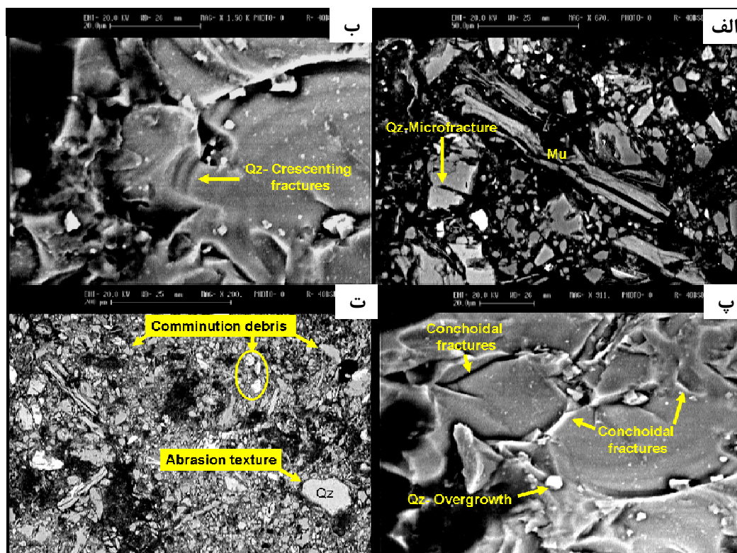
شکل ۵ بافت‌های سطحی کانی کوارتز (Qz) در نهشته‌های بادرفتی استان گلستان با استفاده از میکروسکوپ الکترونی روبشی (SEM). (الف): بافت ریز شکستگی (Microfracture texture) و حضور چند رشته تار مسکویت (Mu)، (ب): شکستگی‌های موازی هلالی شکل Crescenting (fractures)، (پ): شکستگی‌های صدفی (Conchoidal fractures) و گرهک‌های بلورین با بافت بر رشدی (Overgrowth)، و (ت): بافت سایشی (Abrasion texture) و واریزه های خردشدگی کوارتز (Comminution debris).
