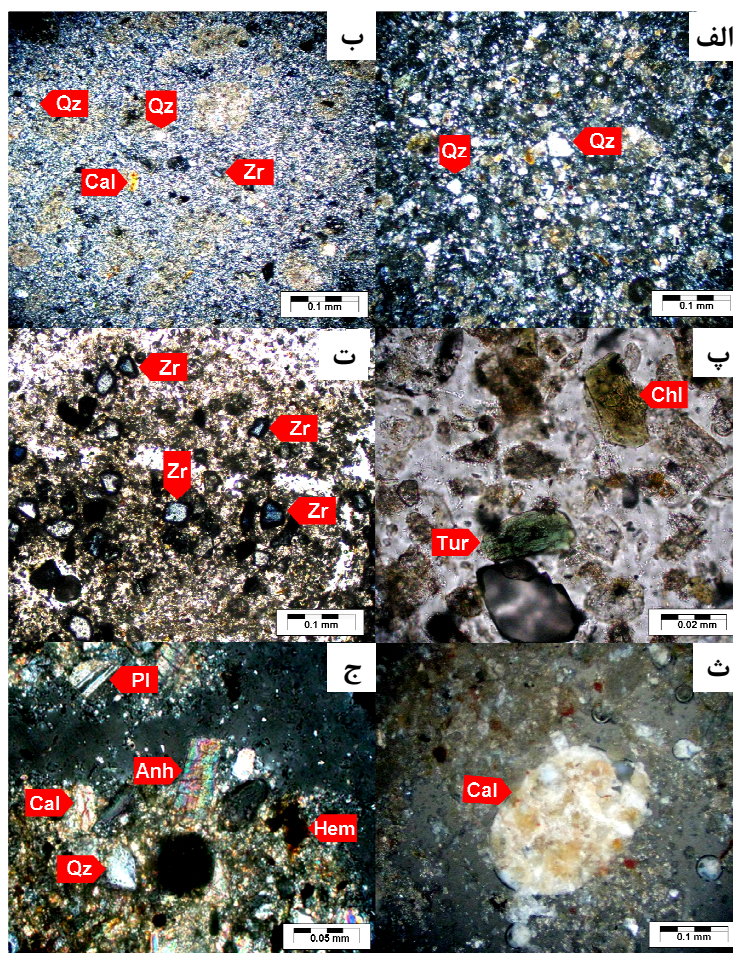
شکل ۲ (الف): فراوانی کوارتزهای درشت دانه (Qz) در حد ماسه خیلی ریز دانه تا سیلت درشت دانه (۰/۰۳۱-۰/۱۲۵ میلی‌متر) در مقاطع شمال شرقی (XPL)؛ (ب): کاهش اندازه ی ذرات تشکیل دهنده بادرفت‌ها در حد سیلت میان دانه تا رس (۰/۰۳۹-۰/۰۱۵۶ میلی‌متر) در مقاطع جنوب غربی (کوارتز (Qz) + زیرکن (Zr) + کربنات کلسیم (Cal) (XPL)؛ (پ): درشت بلور تورمالین (Tur) + کلریت منیزیم دار (Chl) (PPL)؛ (ت): زیرکن‌های درشت دانه (Zr) با حاشیه متامیکتی در مقاطع شمال شرق (PPL)؛ (ث): کربنات کلسیم (Cal) با بافت هسته ریخت (Cytomorphic) (XPL) و (ج): انیدریت (Anh) + پلاژیوکلاز (Pl) + هماتیت (Hem) + کربنات کلسیم (Cal) (XPL).
