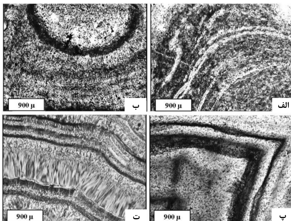
شکل ۴ بافت‌های میکروسکوپی در سنگ‌های ایگنیمبریتی و آگات‌های منطقه‌ی میانه: (الف) بافت جریان (ppl) (ب) بافت اسفرولیتی (ppl) (پ) بافت نواری (xpl) (ت) بافت رشته‌ای (xpl).
