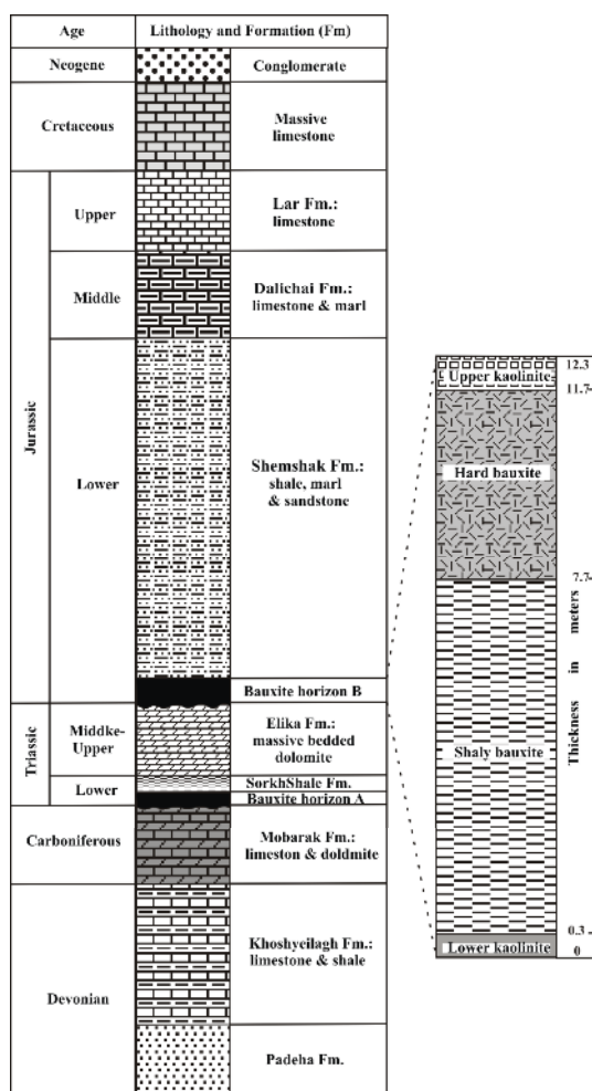
شکل ۲ دنباله‌ی چینه‌شناسی شماتیک واحدهای سنگ‌چینه‌ای موجود در منطقه‌ی جاجرم (چپ). افق بوکسیتی B واقع در بخش گل‌بینی. این نیمرخ یکی از نیمرخ‌های مورد بررسی در این پژوهش است [۲۰-۲۲].
