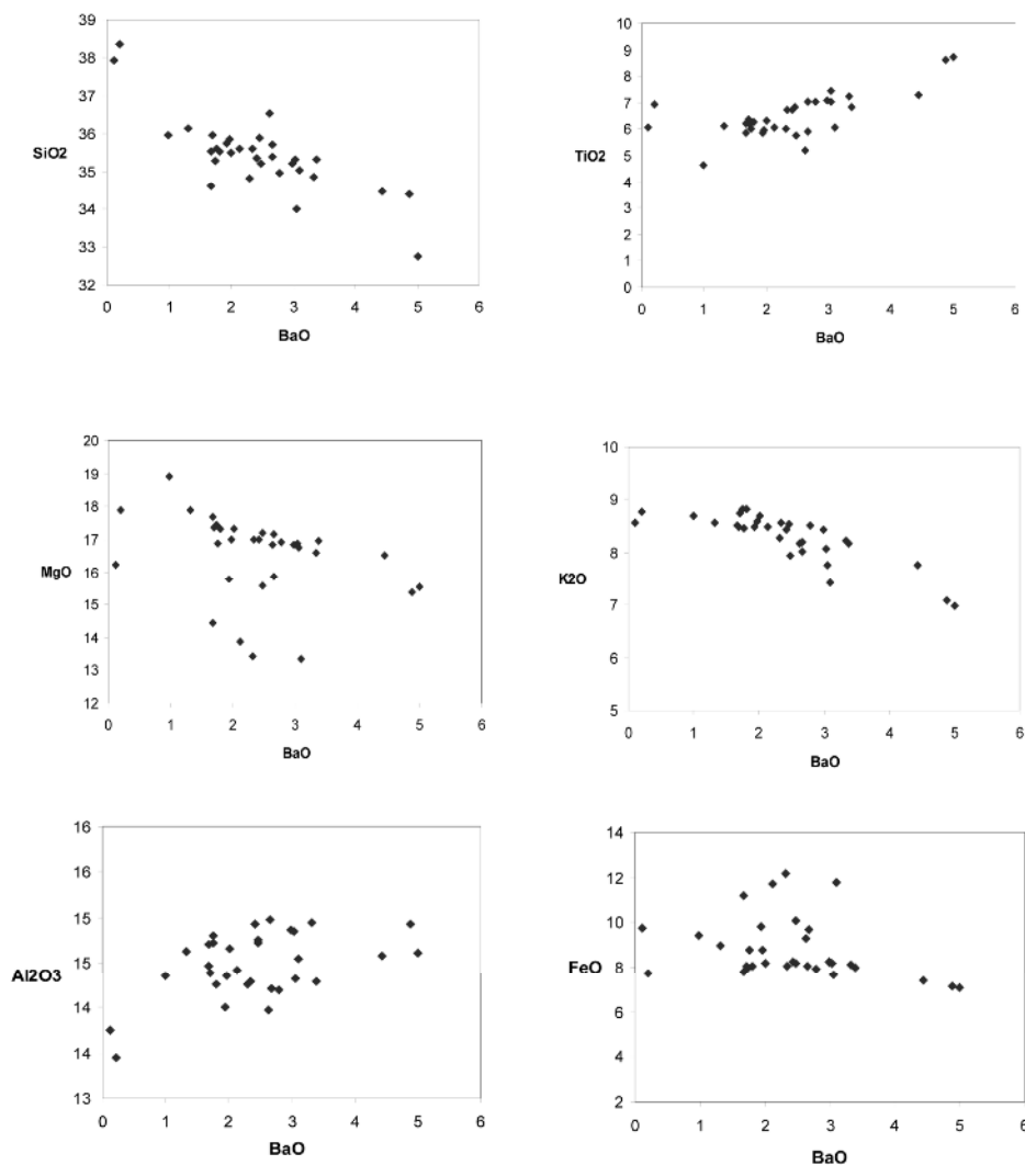
شکل ۳ نمودار تغییرات BaO نسبت به اکسیدهای \text{TiO}_2 , \text{SiO}_2 , \text{MgO} , \text{K}_2\text{O} , \text{FeO} , \text{Al}_2\text{O}_3 و \text{BaO} همبستگی مثبت بین \text{TiO}_2 , \text{Al}_2\text{O}_3 و \text{BaO} و همبستگی منفی با اکسیدهای \text{SiO}_2 , \text{MgO} , \text{K}_2\text{O} , \text{FeO} مشاهده می‌شود.
