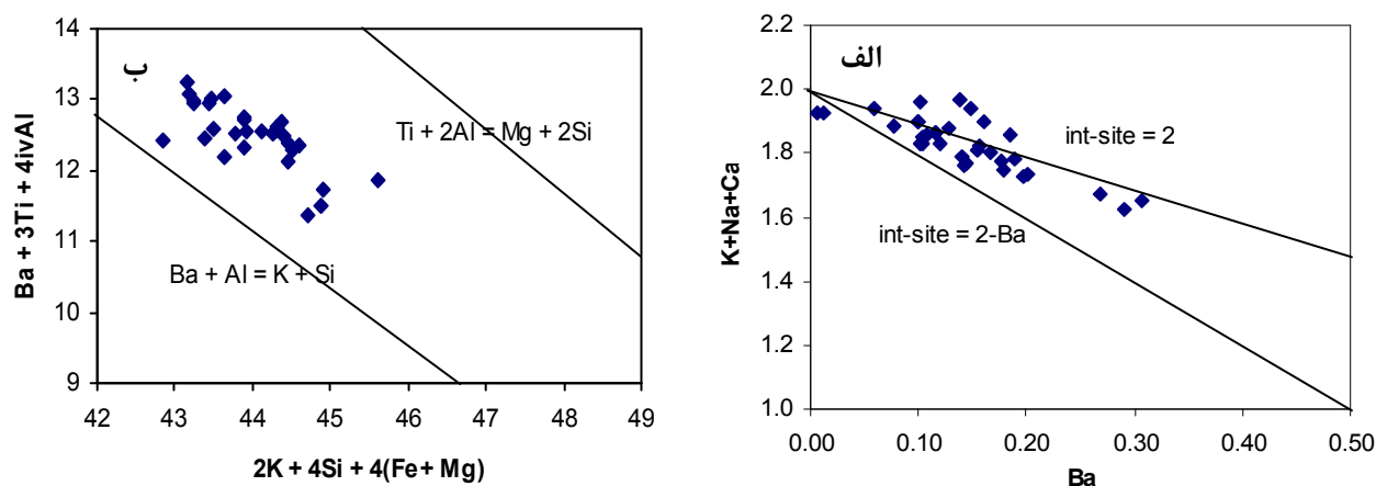
شکل ۴ الف) نشستن باریم به جای کاتیون‌های بین لایه‌ای در نمونه‌های بررسی شده، ب) نمودار 2\text{K} + 4\text{Si} + 4(\text{Fe} + \text{Mg}) نسبت به \text{Ba} + 3\text{Ti} + 4\text{ivAl} برای نشان دادن روند زوج جایگزینی \text{Ba} + \text{Al} = \text{K} + \text{Si} در فلوگوپیت‌های بررسی شده [۸].
