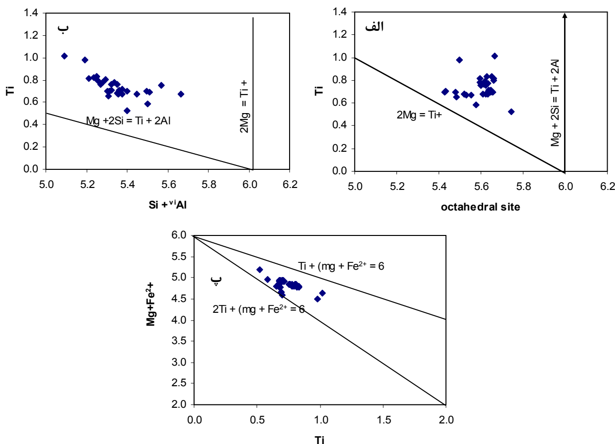
شکل ۵ جایگزینی Ti در موقعیت‌های هشت وجهی (الف) نمودار Ti نسبت به مجموع کاتیون‌های موقعیت هشت وجهی (ب) نمودار Ti نسبت به + SiAl^{VI} (پ) نمودار Ti نسبت به (Mg + Fe^{2+}) نمودارهای الف و ب از [۱۵] و نمودار پ از [۲].
