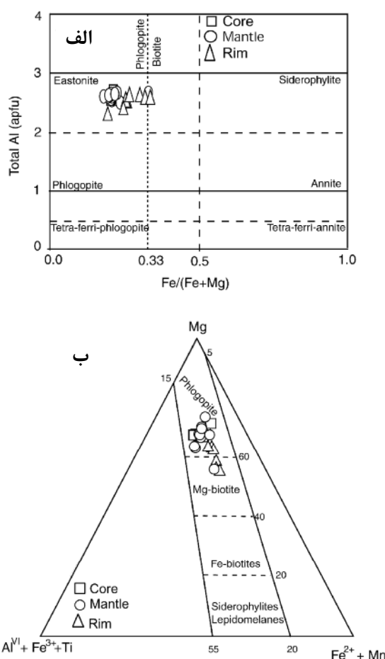
شکل ۲ الف) ترکیب میکاهای بررسی شده در نمودار رده‌بندی میکاها بر اساس [۷]، ب) نمونه‌های بررسی شده در نمودار Mg-(Al^{VI} + Fe^{3+} + Ti)-(Fe^{2+} + Mn) در گستره‌ی فلوگوپیت قرار می‌گیرند.
