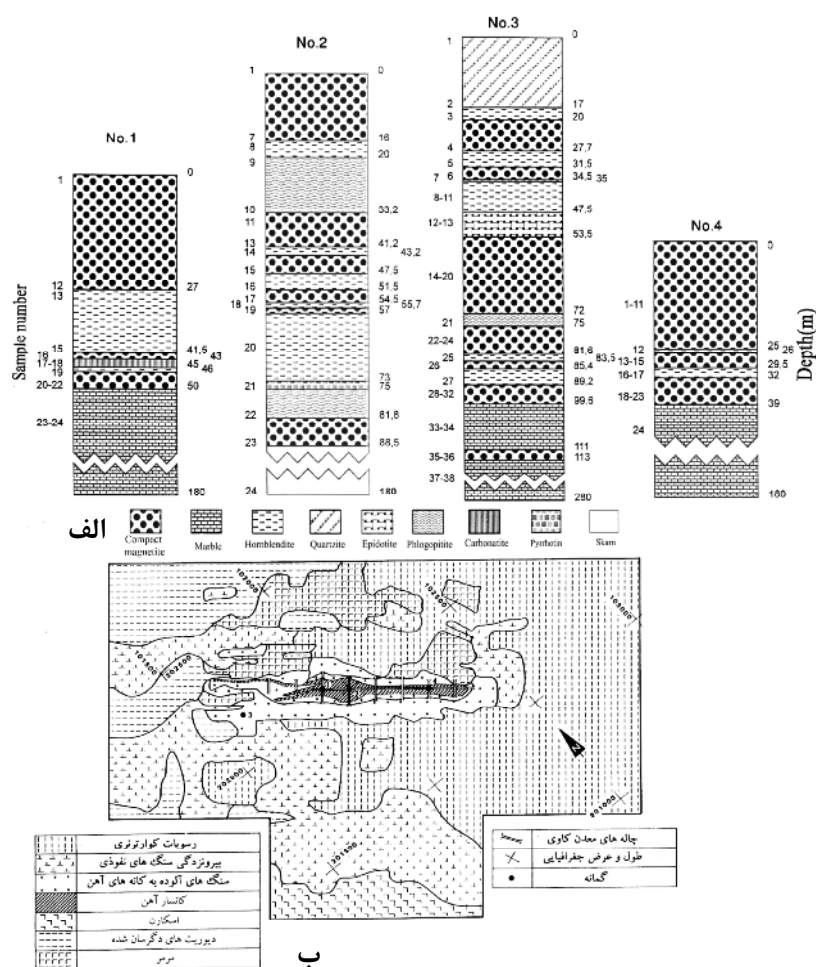
شکل ۲ الف) نیم‌رخ گمانه‌های ۱، ۲، ۳ و ۴ (ب) موقعیت چاله‌های معدن‌های کوهی در نقشه‌ی زمین‌شناسی کانسار گلالی [۱۰] (ب‌تغییرات).
