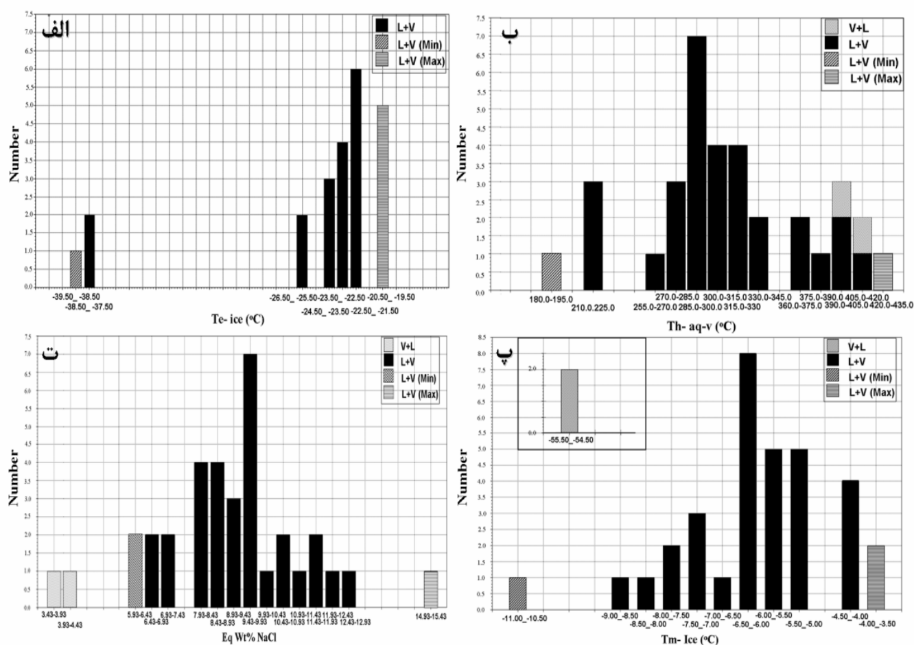
شکل ۶ نمودارهای ستونی میانبارهای شاری. الف: دمای ذوب اولین قطعه یخ یا دمای یوتکتیک، ب: دمای همگن شدگی یا یکنواختی، پ: دمای ذوب آخرین قطعه یخ و ت: میزان شوری برحسب درصد وزنی معادل NaCl.
