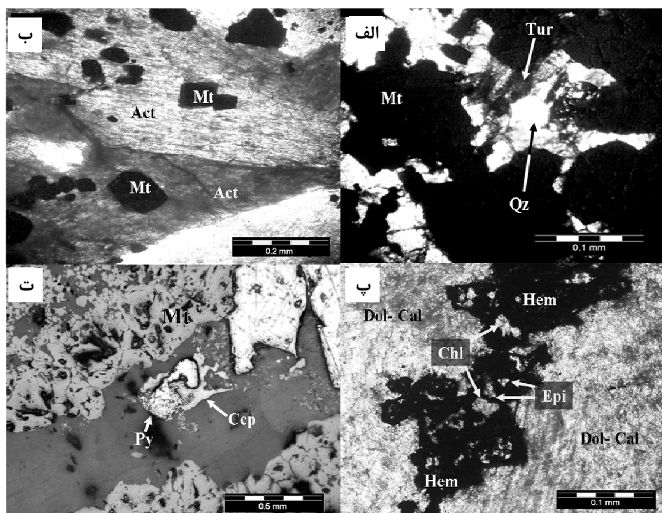
شکل ۴ انواع سیلیکات‌ها و سولفیدهای همراه با اکسیدهای آهن در نور متقاطع (XPL)، طبیعی (PPL) و بازتابی (RL). (الف): پاراژنز مگنتیت-کوارتز-تورمالین (Tur)، (XPL) (ب): کانه زایی مگنتیت همراه با اکتینولیت، (PPL) (پ): کلریت (Chl)-اپیدوت (Epi) همراه با کانه‌زایی هماتیت (XPL) و (ت): فازهای تاخیری پیریت (Py) + کلکوپیریت (Ccp) در مگنتیت (RL).
