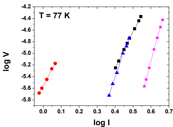
شکل ۸ نمودار \log V - \log I برای نمونه‌های آلاینش داده شده با مقادیر مختلف نانوذرات طلا (■) ۰٫۱٪، (●) ۰٫۵٪، (★) ۱٪ و (▲) ۲٪ با زمان پخت ۷۲ ساعت.
