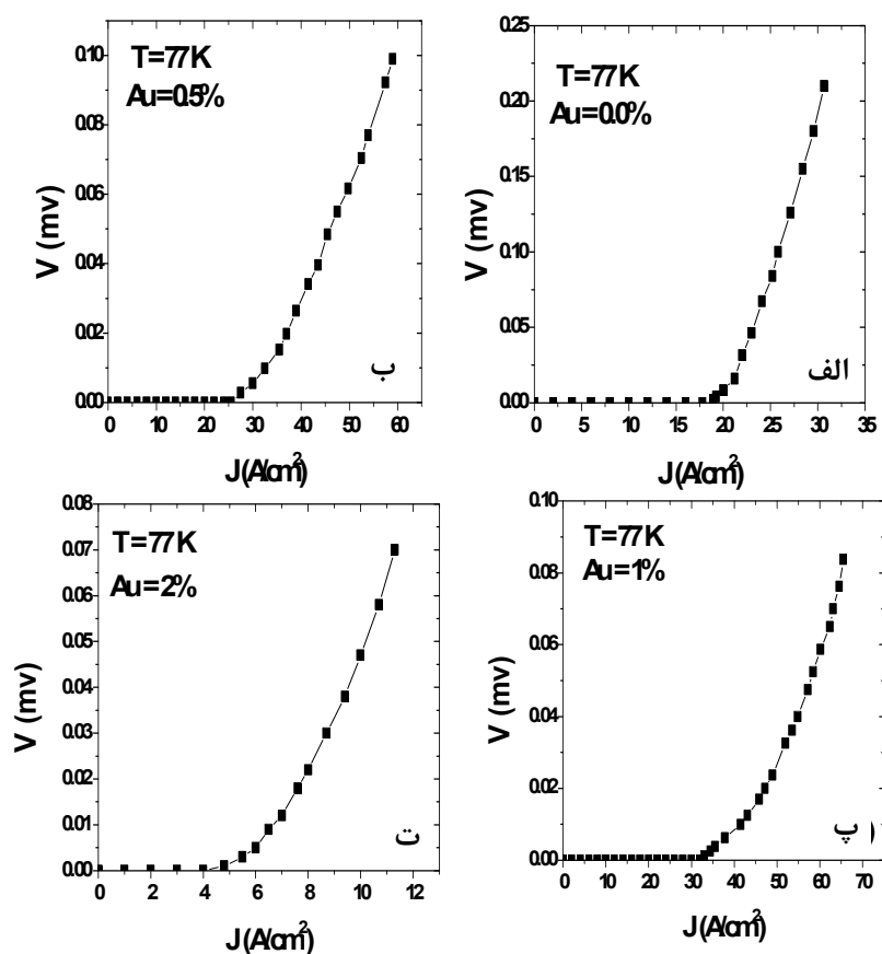
شکل ۵ نمودارهای V-I برای مقادیر متفاوت نانوذرات طلا (الف، ۰/۰٪، ب، ۰/۵٪، ج، ۱٪، د، ۲٪) با زمان پخت ۷۲ ساعت.
