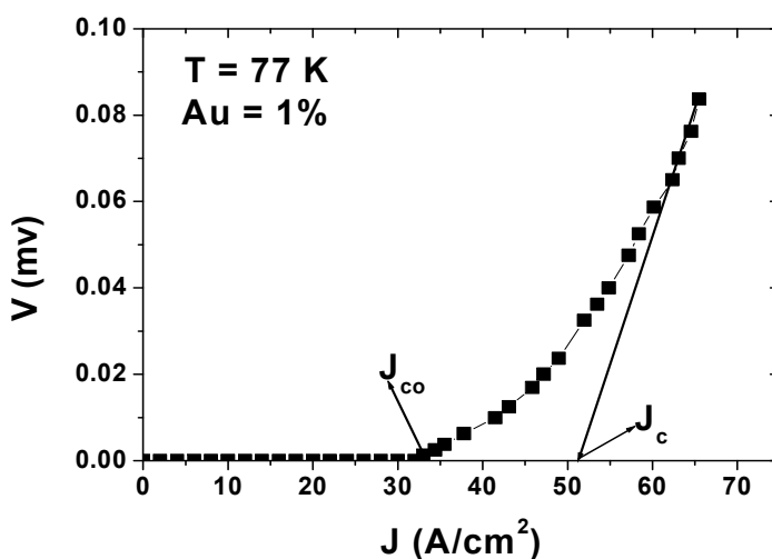
شکل ۷ نمودار V-J برای نمونه‌ی آلاینش داده شده با نانوذرات طلا به مقدار ۱٪ با زمان پخت ۷۲ ساعت.
