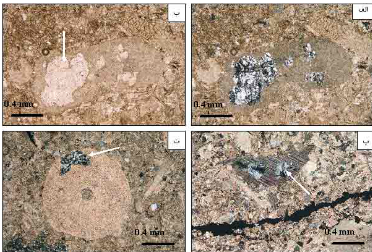
شکل ۳ الف) سیلیسی شدن بلورهای منفرد اکتینودرم (XPL) (ب) تصویر الف در PPL که بلور منفرد اکتینودرم با حفره پر شده به وسیله سیلیس در آن بهتر تشخیص داده می‌شود. (پ) خرده اکتینودرم که در سطوح ضعیف رخ آن کوارتز کلسدونی جانشین شده است (XPL). (ت) سیلیسی شدن به شکل کوارتز دانه‌ای در خرده اکتینودرم (XPL).
