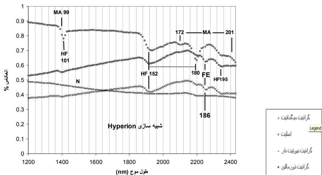
شکل ۱۰ شبیه سازی طیف‌های چند نمونه سنگ پرونزد بر اساس عملکرد سنجنده فراطیفی Hyperion.
