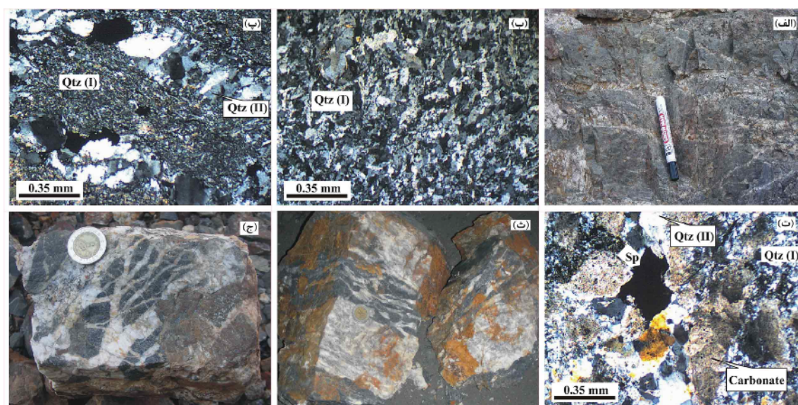
شکل ۴ تصاویر صحرایی و میکروسکوپی از دگرسانی سیلیسی و برشی شدن در کانسارهای عمارت و موچان الف) سنگ آهک به شدت سیلیسی شده در کانسار عمارت؛ ب) سیلیسی شدن مرحله اول در کانسار عمارت که باعث جانشینی کامل سنگ آهک با کوارتز شده است؛ پ) سیلیسی شدن مرحله دوم در کانسار عمارت که با وجود رگچه های کوارتزی در سنگ میزبان سیلیسی شده مشخص می شود؛ ت) سیلیسی شدن مراحل اول و دوم همراه با کانی سازی اسفالریت و کربنات های جانشین نشده در کانسار موچان؛ ث) برش انحلالی در کانسار عمارت؛ ج) برش گرمایی در کانسار موچان. اختصارات: Qtz (I): کوارتز مرحله اول، Qtz (II): کوارتز مرحله دوم، Sp: اسفالریت، Gn: گالن. تصاویر میکروسکوپی در با استفاده از نور قطبیده گرفته شده است.
