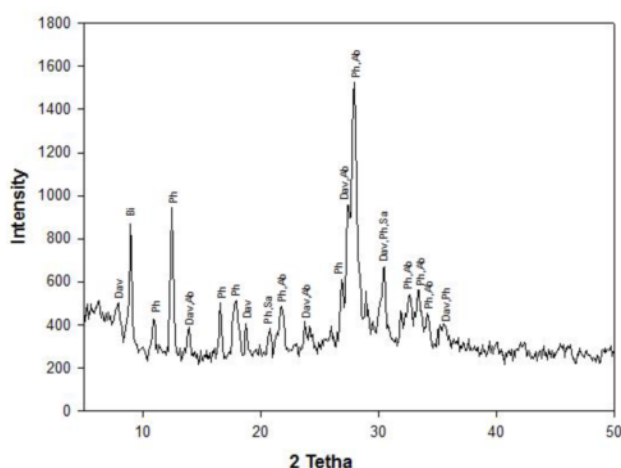
شکل ۲ الگوی XRD نمونه سنتزی TN 5 . در این نمونه از غلظت ۵ مول بر لیتر برای هر دو نوع آبگون پتاس و نمک طعام استفاده شد. Bi: بیوتیت، Sa: سانیدین، Ab: آلپیت، Ph: فیلپسیت و Dav: هیدروکسی داوین.
