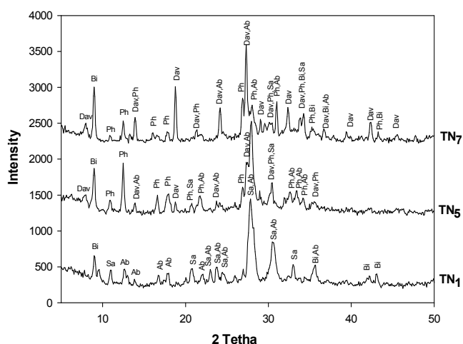
شکل ۴ مقایسه‌ی الگوهای پراش پرتو ایکس نمونه‌های سنتزی TN_5 و TN_7 با الگوی XRD نمونه‌ی اولیه ( TN_1 ). در این نمونه‌ها از آبگون‌های KOH و NaCl در غلظت‌های یکسان ۵ مول بر لیتر برای نمونه‌ی TN_5 و نیز به ترتیب در غلظت‌های ۷٫۵ مول بر لیتر و ۲٫۵ مول بر لیتر برای نمونه‌ی TN_7 استفاده شده است. Bi: بیوتیت، Sa: ساندین، Ab: آلبیت، Ph: فلیپسیت و Dav: هیدروکسی‌داوین.
