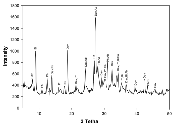
شکل ۳ الگوی XRD نمونه‌ی سنتزی TN_7 . در این نمونه از آبگون‌های با غلظت ۷٫۵ مول بر لیتر برای پتاس و ۵ مول بر لیتر برای نمک طعام استفاده شده است. Bi: بیوتیت، Sa: سانیدین، Ab: آلیت، Ph: فلیسیت و Dav: هیدروکسی‌داوین.
