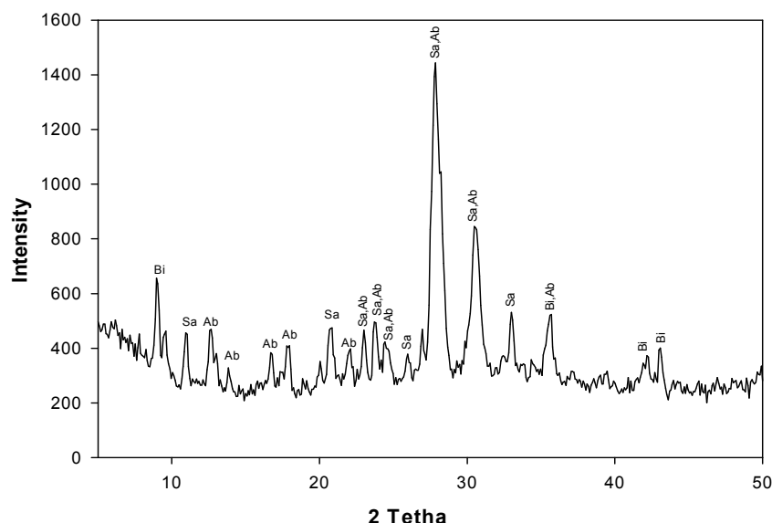
شکل ۱ الگوی پراش پرتو ایکس (XRD) نمونه اولیه (TN 1 ): بیوتیت، Sa: سانییدین و Ab: آلبیت.
