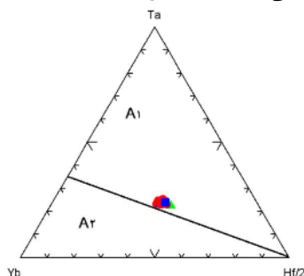
ت- نمودار سه تایی Yb-Ta-Hf/2 از [۶]
