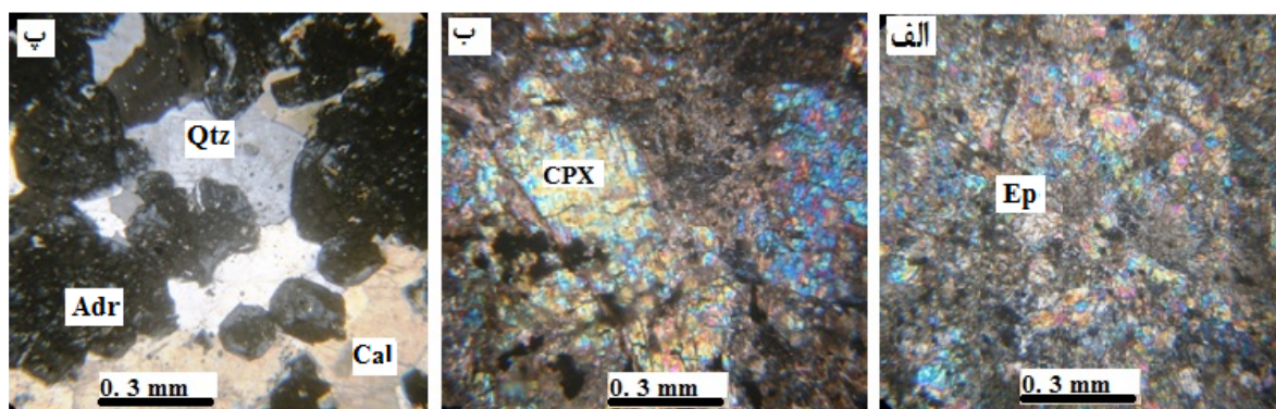
شکل ۴. تصویر میکروسکوپی از کانی‌های اسکارن در نور XPL. (الف) اپیدوت (Ep) با رنگ تداخلی متغیر. (ب) بلورهای کلینوپیروکسن (Cpx) دگرسان شده (پ) بلورهای گارنت (Adr) در زمینه‌ای از کوارتز (Qz) و کلسیت (Cal) اقتباس از [۶].
