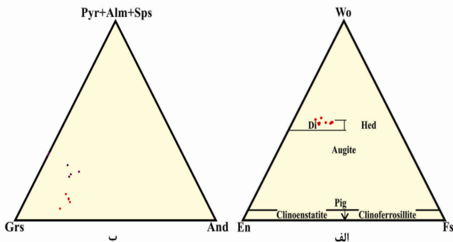
شکل ۳ الف) موقعیت ترکیب کلینوپیروکسن‌های اسکارن قروه در نمودار مثلثی طبقه بندی پیروکسن‌ها [۶]. ب) موقعیت ترکیب گارنت‌های اسکارن قروه در نمودار مثلثی طبقه بندی گارنت‌ها [۳۰].
